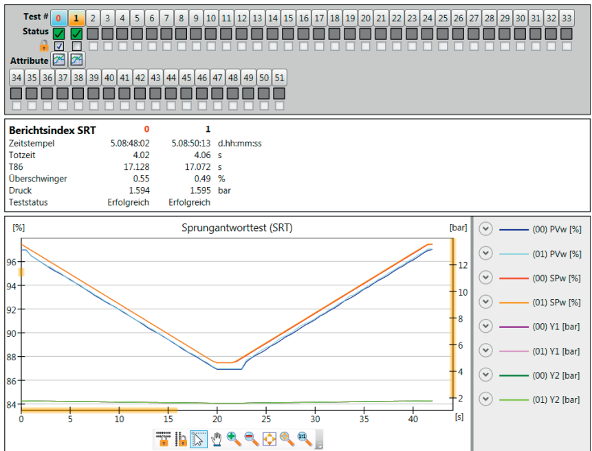
Bild 8: Sprungantworttest (PST)
