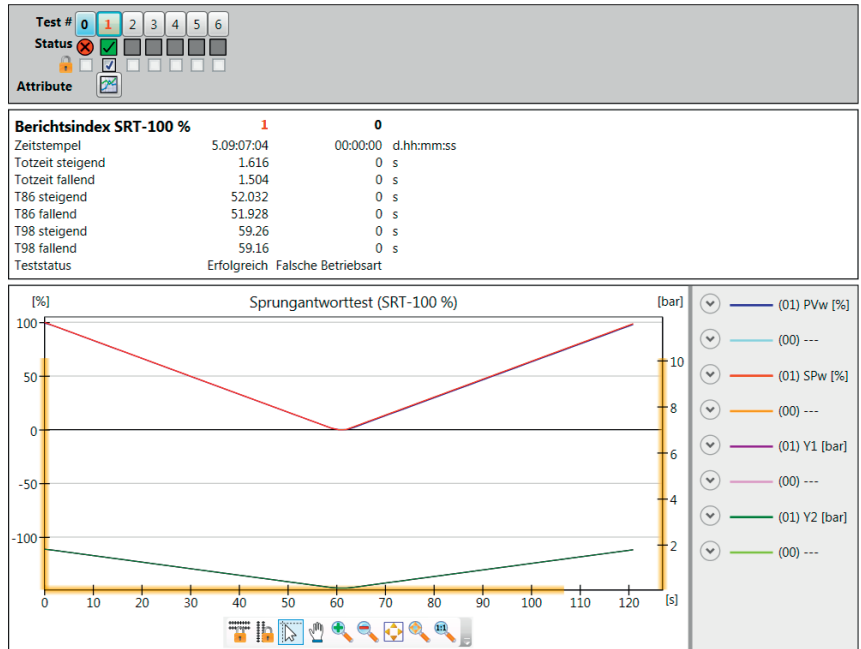
Bild 9: Sprungantworttest (FST)
