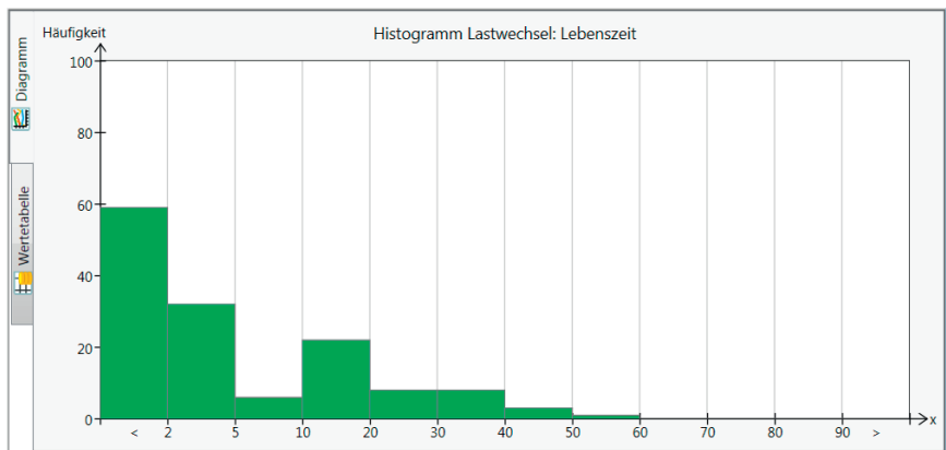
Bild 6: Histogramm Lastwechsel
