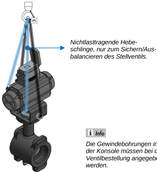
Bild 5.9: Hebepunkte - DKV Baureihe 72.4/AT
