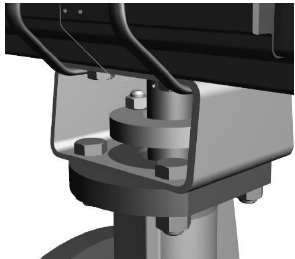
Bild 7.2: Detail A · Befestigung der Hebeschlingen am Bügel
