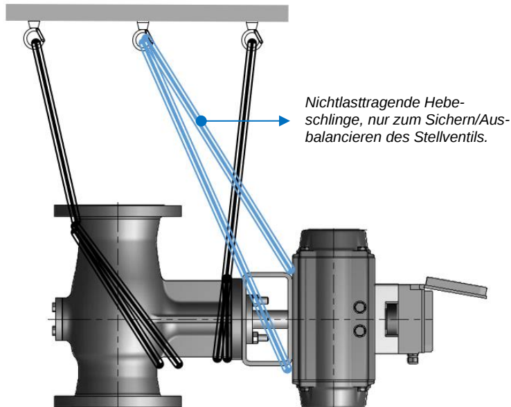
Bild 5.8: Hebepunkte - DKV Baureihe 72/AT, 73/AT, 82/AT
