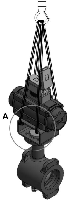
Bild 5.12: Hebepunkte - DKV Baureihe 72.4/AT
