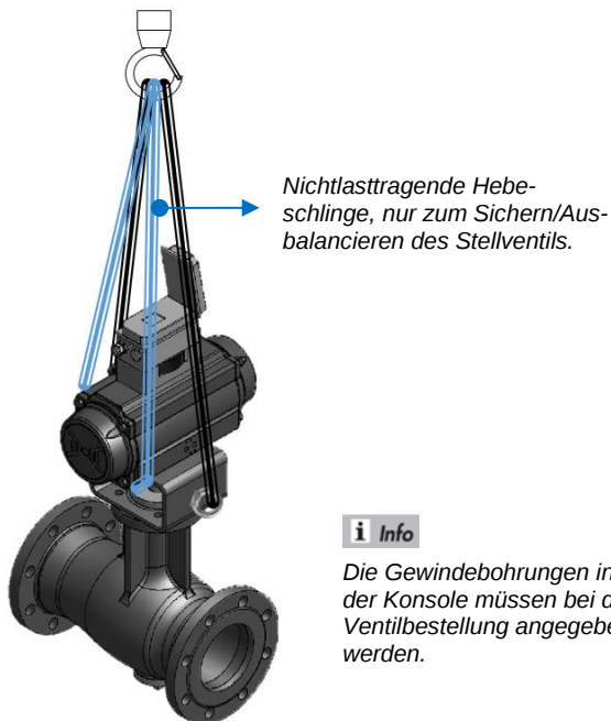
Bild 5.3: Hebepunkte - DKV Baureihe 72/AT, 73/AT, 82/AT
