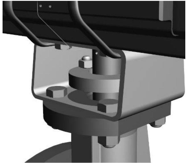
Bild 5.13: Detail A · Befestigung der Hebeschlingen am Bügel
