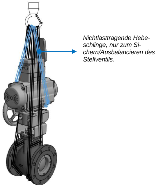
Bild 6. 1: Hebepunkte - DKV Baureihe 72/AT, 73/AT, 82/AT
