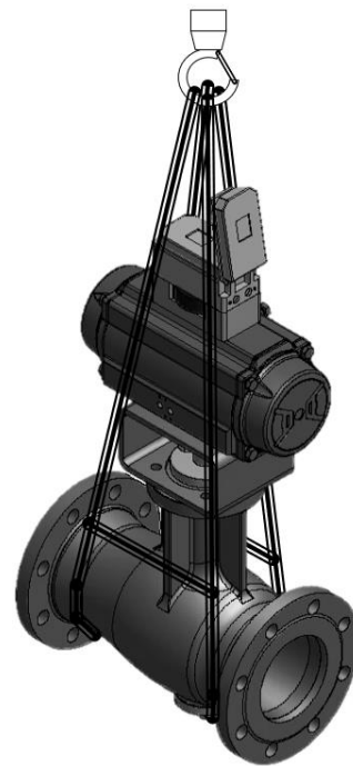
Bild 5.2: Hebepunkte - DKV Baureihe 72/AT, 73/AT, 82/AT
