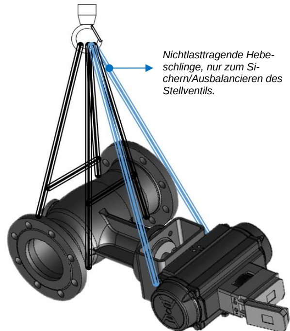
Bild 5.4: Hebepunkte - DKV Baureihe 72/AT, 73/AT, 82/AT
