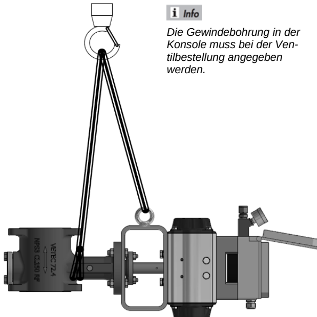
Bild 5.14: Hebepunkte - DKV Baureihe 72.4/AT
