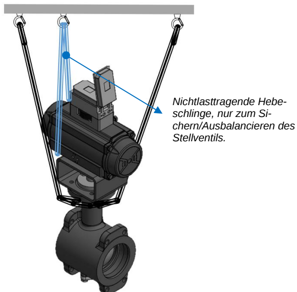
Bild 5.11: Hebepunkte - DKV Baureihe 72.4/AT
