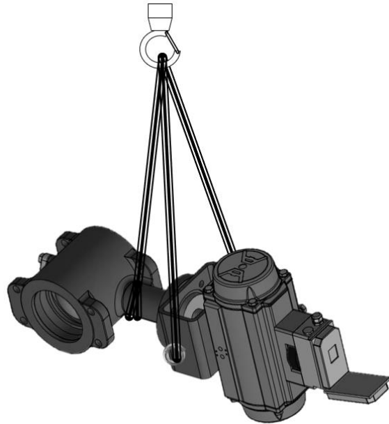
Bild 5.10: Hebepunkte - DKV Baureihe 72.4/AT
