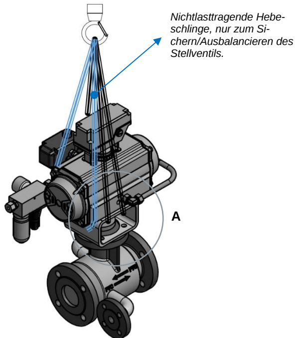
Bild 7.1: Hebepunkte – DKV mit Heizmantel und AT-Antrieb
