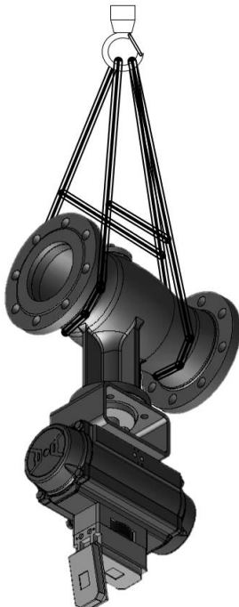
Bild 5.5: Hebepunkte - DKV Baureihe 72/AT, 73/AT, 82/AT
