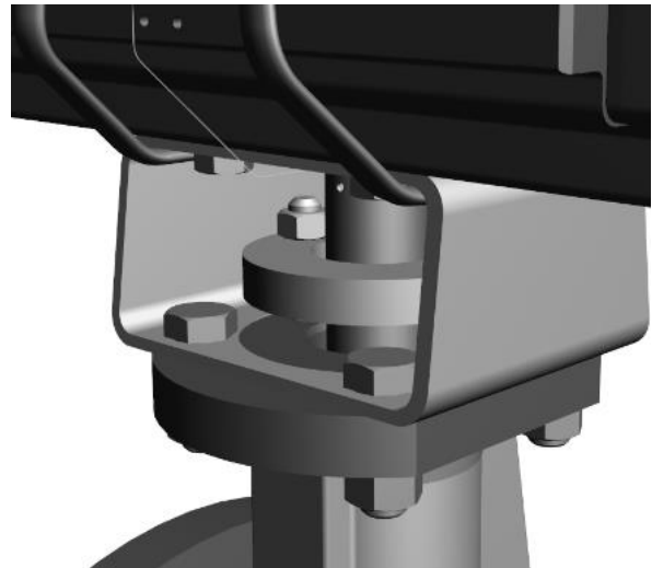
Bild 8.2: Detail A · Befestigung der Hebeschlingen am Bügel
