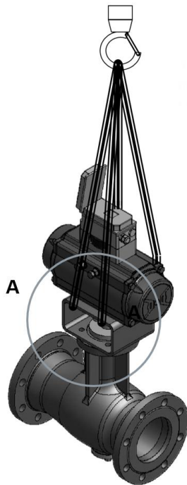
Bild 5.6: Hebepunkte - DKV Baureihe 72/AT, 73/AT, 82/AT
