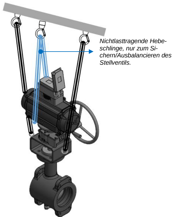
Bild 6. 2: Hebepunkte - DKV Baureihe 72.4/AT
