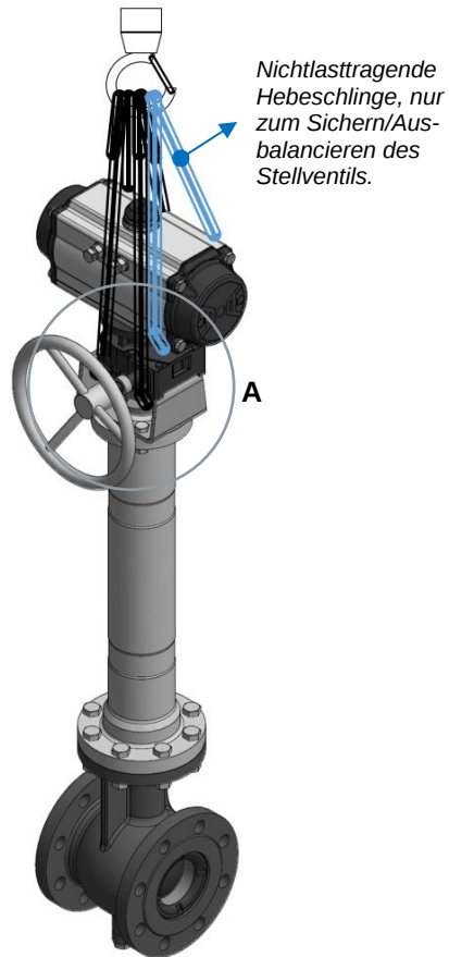
Bild 8.1: Hebepunkte – DKV mit Isolierteil und AT-Antrieb
