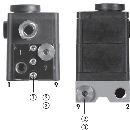
Přípojovací deska
