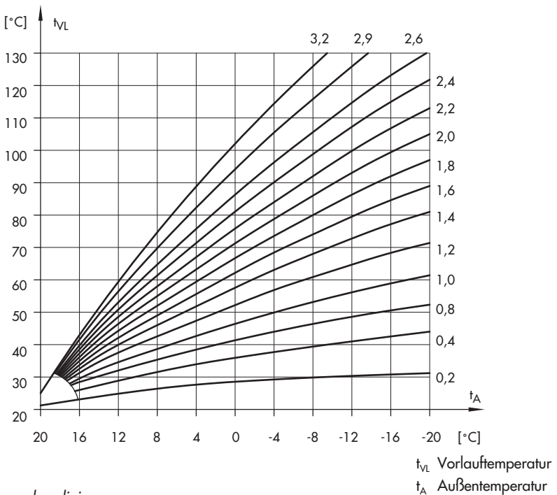
Bild 1 · Steigungskennlinien
