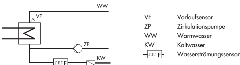
Bild 11 · Aufbau eines Durchflusssystems mit Wasserströmungssensor (CO4 -> F04 - 1, Wahl: AnA)
