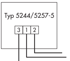
Bild 7 · Anschlussplan Raumleitgerät Typ 5244/5257-5 an TROVIS 5575 für Rk1 oder Rk2
