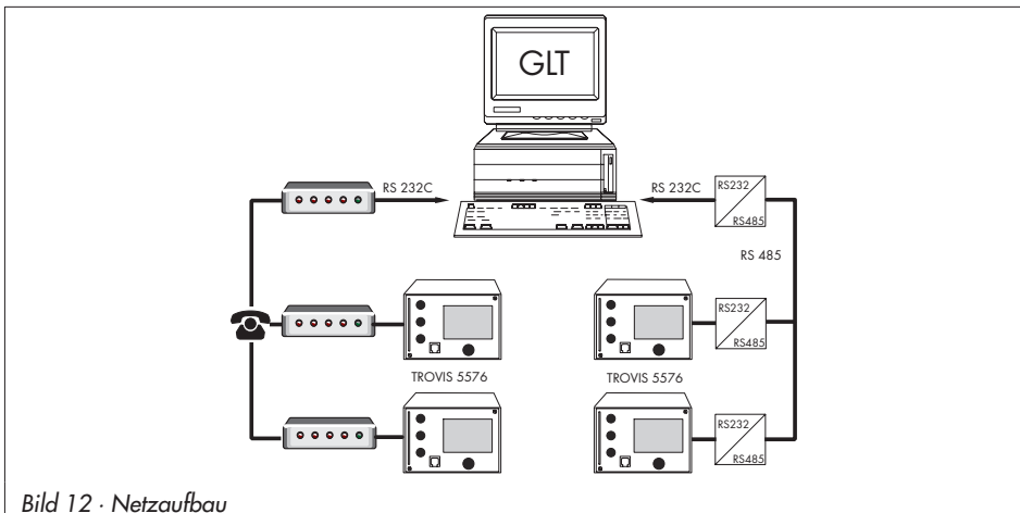
Bild 12 · Netzaufbau
