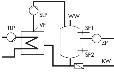
Bild 10 · Aufbau eines Speicherladesystems
