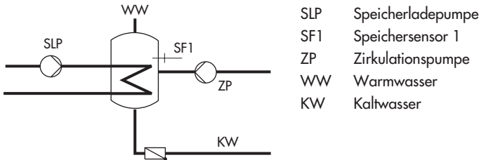
Bild 8 · Aufbau eines Speichersystems
