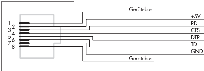
Bild 14 · Belegung der RJ 45-Anschlussbuchse
