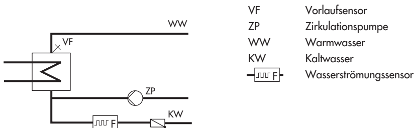
Bild 11 · Aufbau eines Durchflusssystems mit Wasserströmungssensor (CO4 -> F04 - 1, Wahl: AnA)
