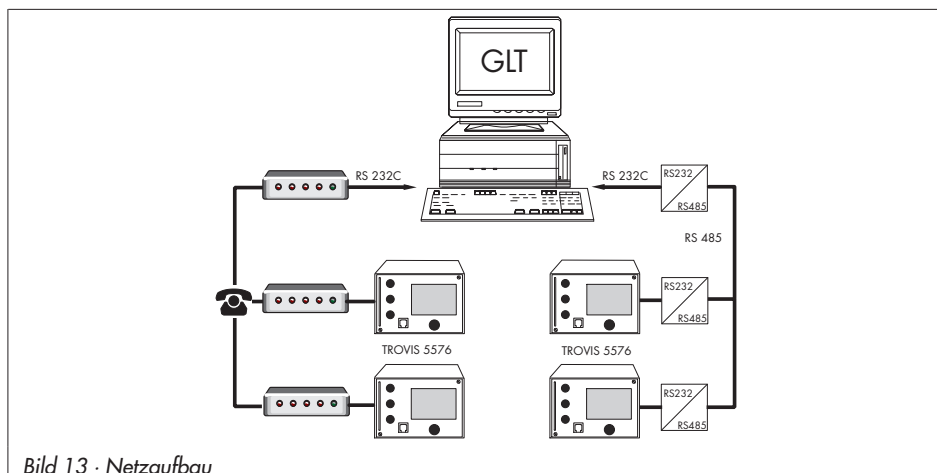
Bild 13 · Netzaufbau
