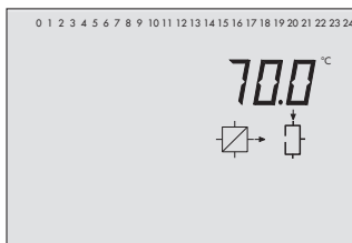
Vorlaufsensor VF4
