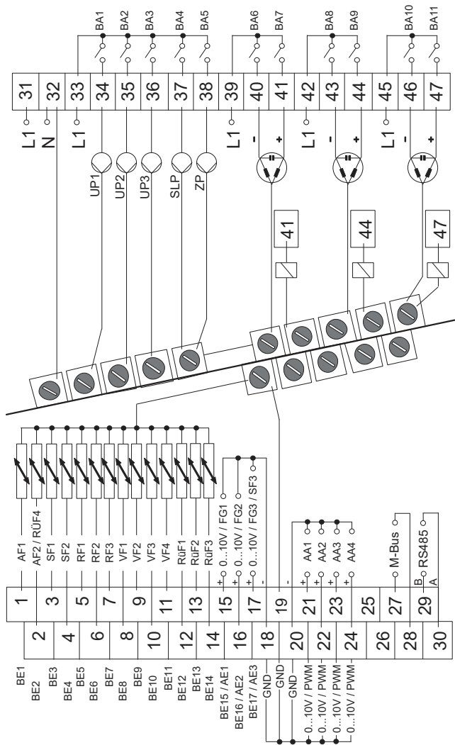
Bild 5-2: Elektrischer Anschluss des Heizungs- und Fernheizungsreglers TROVIS 5578-1113
