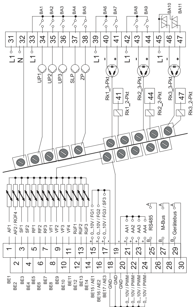
Bild 5-3: Elektrischer Anschluss des Heizungs- und Fernheizungsreglers TROVIS 5578-1114
