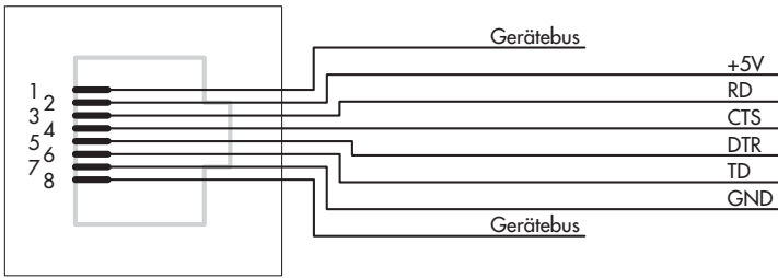
Bild 12 · Belegung der RJ 45-Anschlussbuchse
