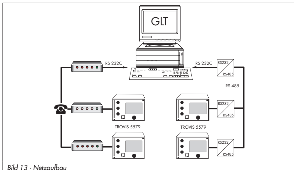
Bild 13 · Netzaufbau
