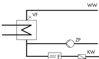
Bild 11 · Aufbau eines Durchflusssystems mit Wasserströmungssensor (CO4 -> F01 - 1, Wahl: AnA)
