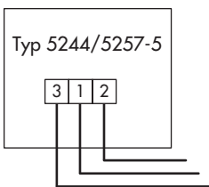
Bild 7 · Anschlüsse Raumleitgerät Typ 5244/5257-5 an TROVIS 5579 für Rk1, Rk2 oder Rk3
