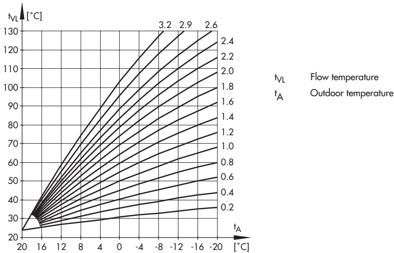
Fig. 5 · Gradient characteristics
