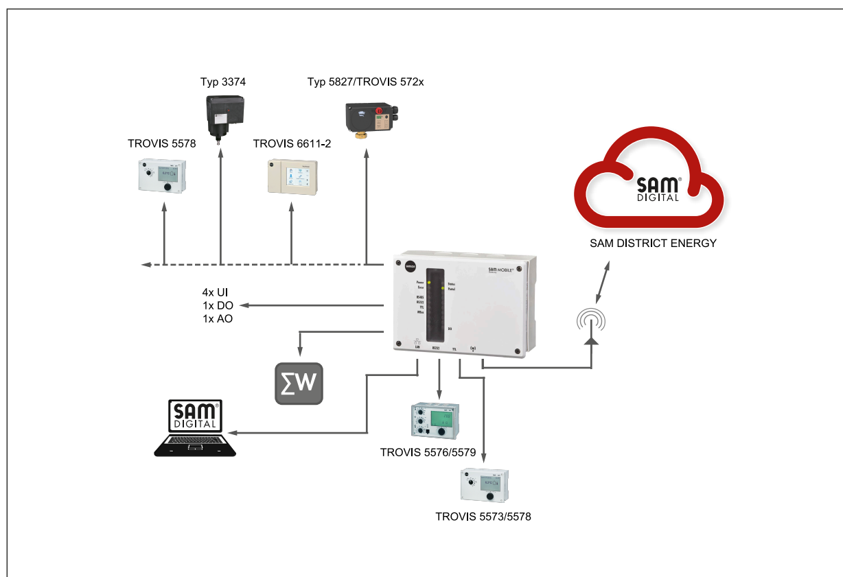
Bild 1: Anwendung des SAM MOBILE+ Gateways
