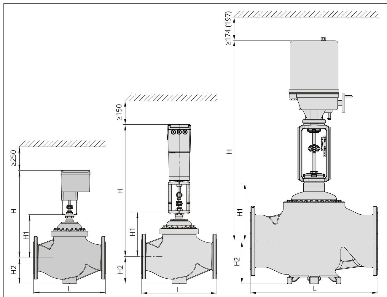
Fig. 4 : Type 3214/3374-10/-11/-21 (à gauche)
