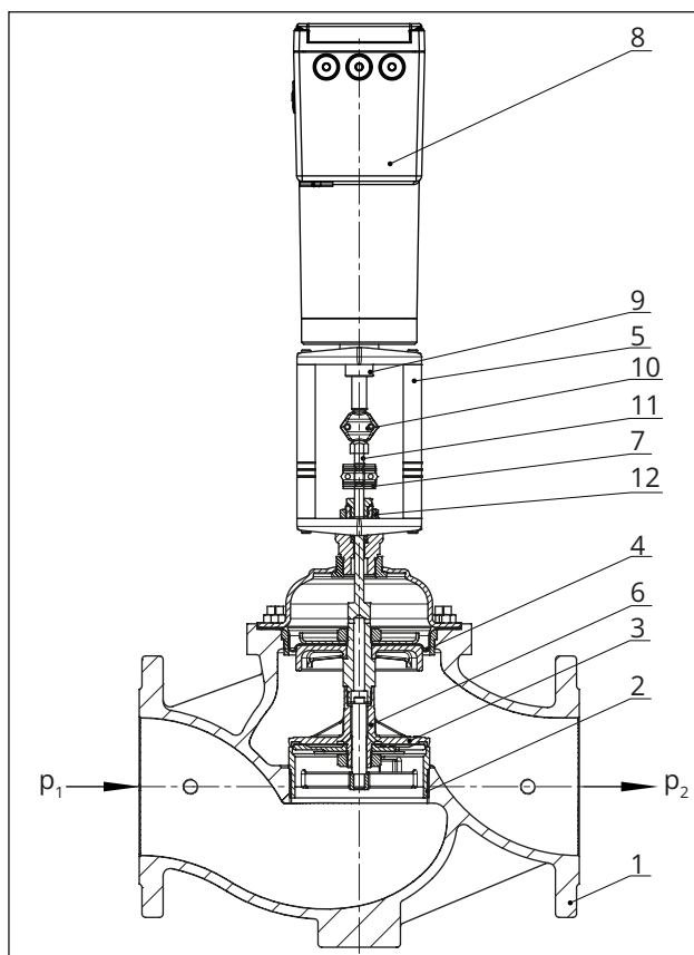
Fig. 3 : Vanne type 3214/3374-27 équilibrée par membrane
