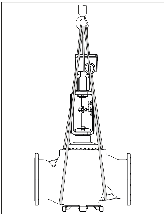
Fig. 5 : Points de levage sur la vanne de régulation
