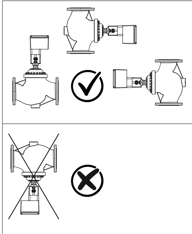
Fig. 6 : Position de montage
