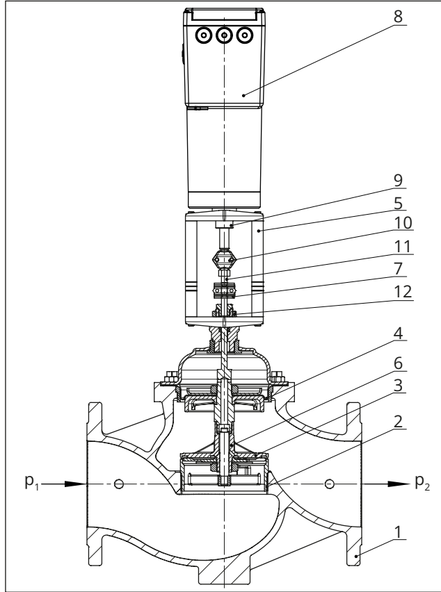
Fig. 7 : Vanne type 3214/3374-27 équilibrée par membrane
