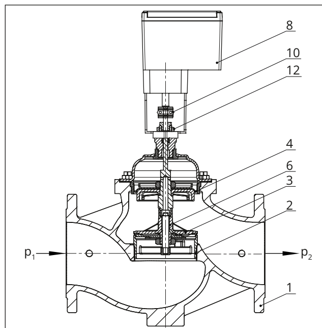
Fig. 2 : Vanne type 3214/3374-10/-11/-21 équilibrée par membrane
