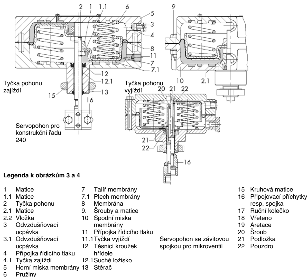
Obr. 3 Servopohony 3271-5 se 120 mm 2 nahoře a 3271-52 se 60 cm 2 dole
