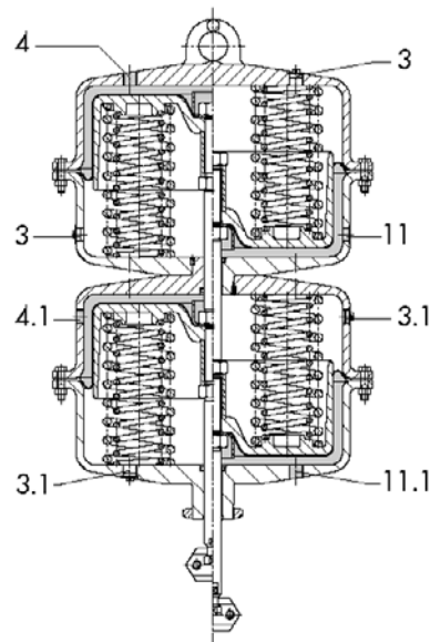
Obr. 4 Tandemový pohon
