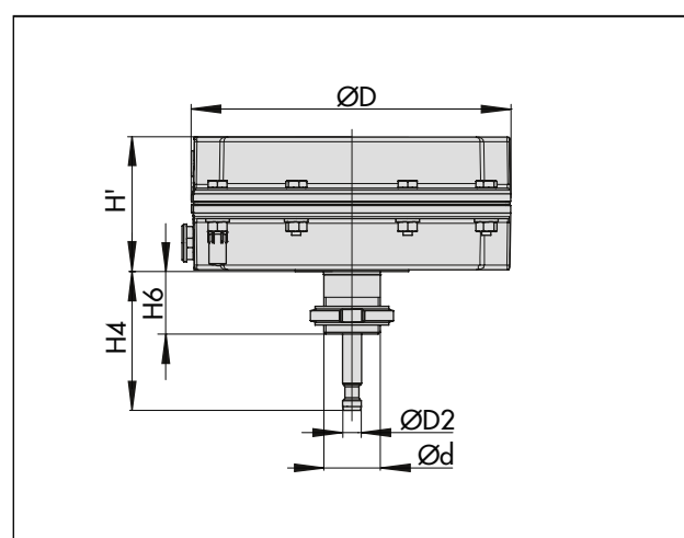
図 7: タイプ 3271-5 ・操作部面積 120 cm 2
