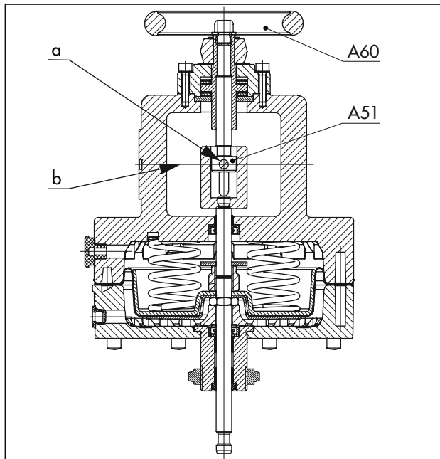
図 17: アクチュエータ タイプ 3271-5、手動ハンドル付き
