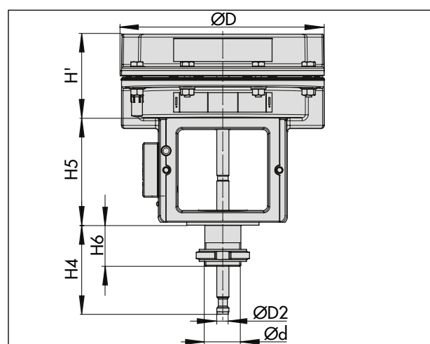
図 9: タイプ 3277-5 ・操作部面積 120 cm 2
