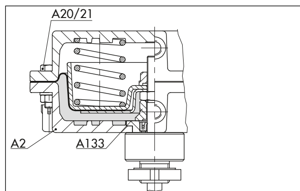
図 3: アクチュエータ タイプ 3271-5 (アクチュエータ軸出)
