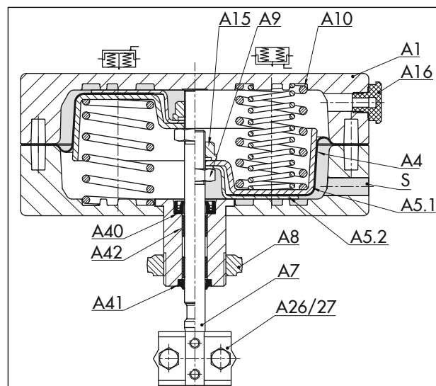
図 2: アクチュエータ タイプ 3271-5 (操作部面積 120 cm 2 の例)
