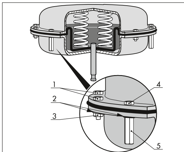
図 22: 事前に荷重がかけられたスプリング（構造図）
