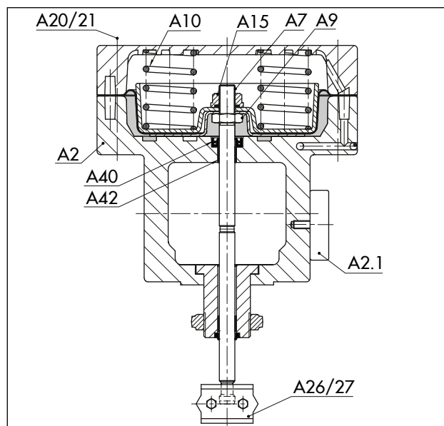
図 4: アクチュエータ タイプ 3277-5、操作部面積 120 cm 2
