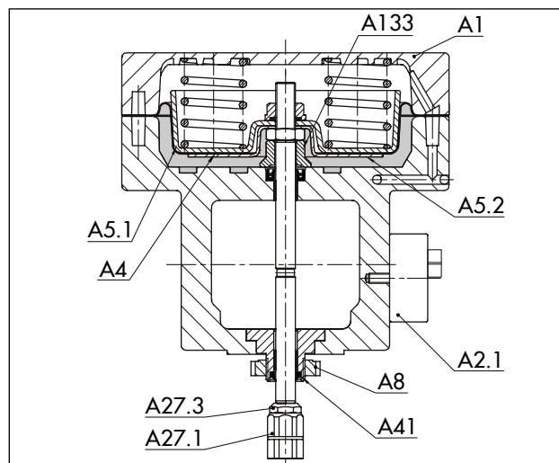
図 5: タイプ 3277-5、マイクロフロー弁 タイプ 3510 への取り付け用
