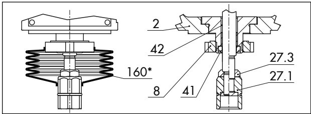
図 24: マイクロフロー弁の仕様への接続
