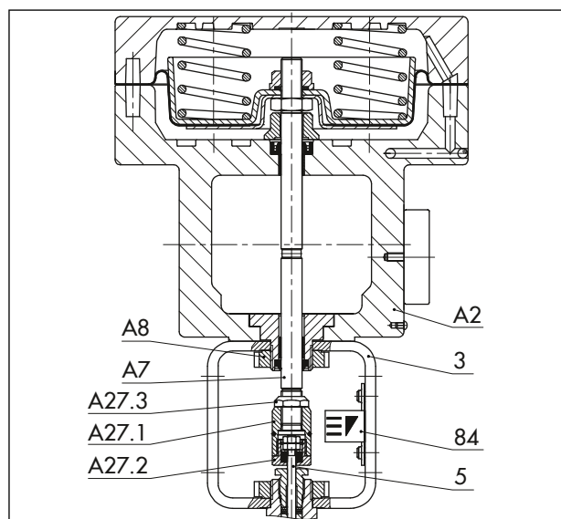
図 21: マイクロフロー弁タイプ 3510 に取り付ける空気式アクチュエータタイプ 3277
