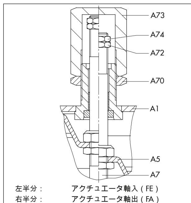
図 16: トラベルストップ
