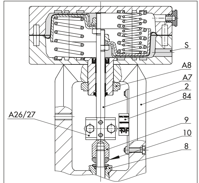
図 12: シリーズ 240 の弁に取り付ける空気式アクチュエータ タイプ 3271
