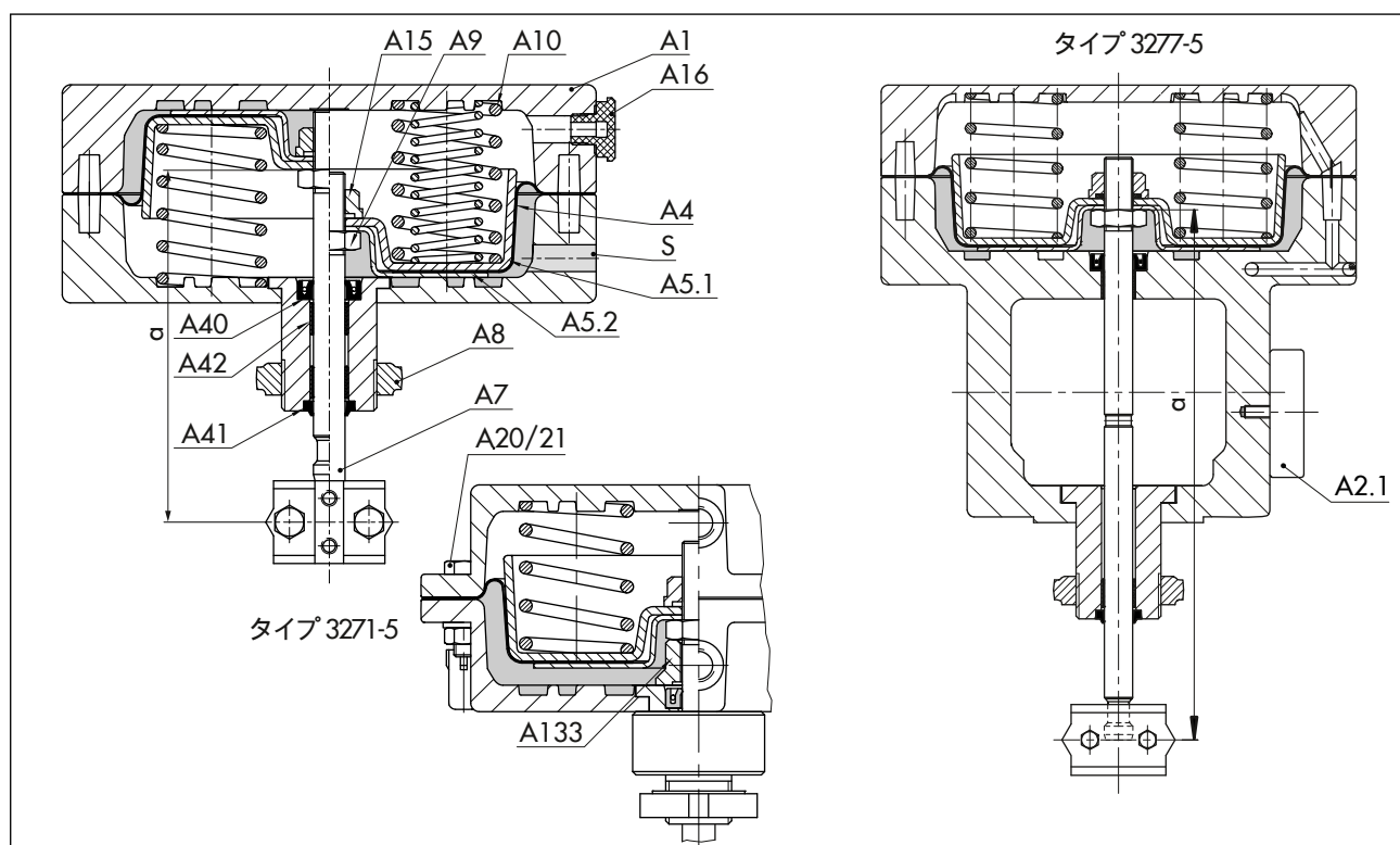
図 18: 空気式アクチュエータ タイプ 3271-5 およびタイプ 3277-5
