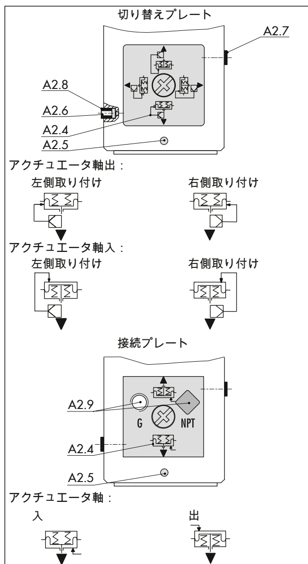
図 6: タイプ 3277-5 の切り替えプレートとコネクティングプレート
