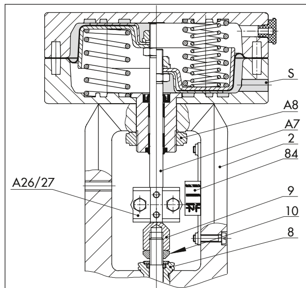
図 20: シリーズ 240 の弁に取り付ける空気式アクチュエータ タイプ 3271
