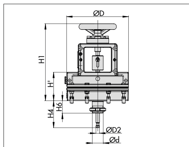
図 8: タイプ 3271-5 追加の手動ハンドル付き
