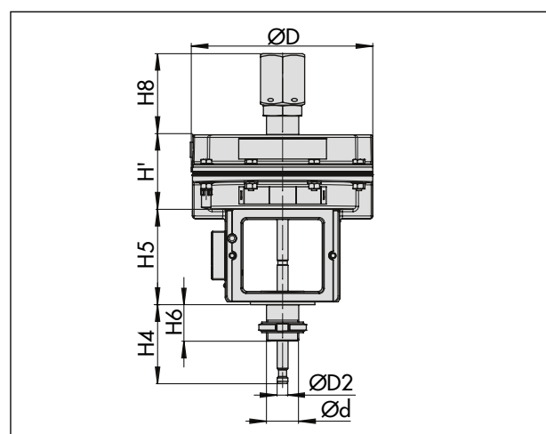
図 10: タイプ 3277-5 トラベルストップ付き
