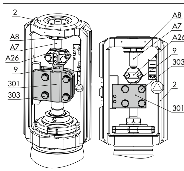
図 14: 回転対策治具：標準仕様（左）と特殊仕様（右）
