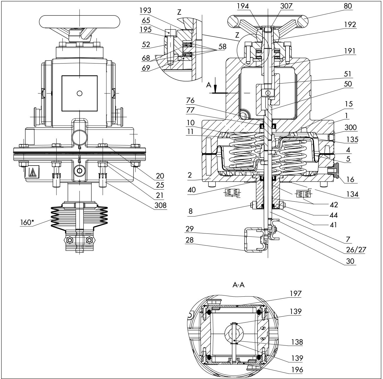
図 23: アクチュエータ タイプ 3271-5
