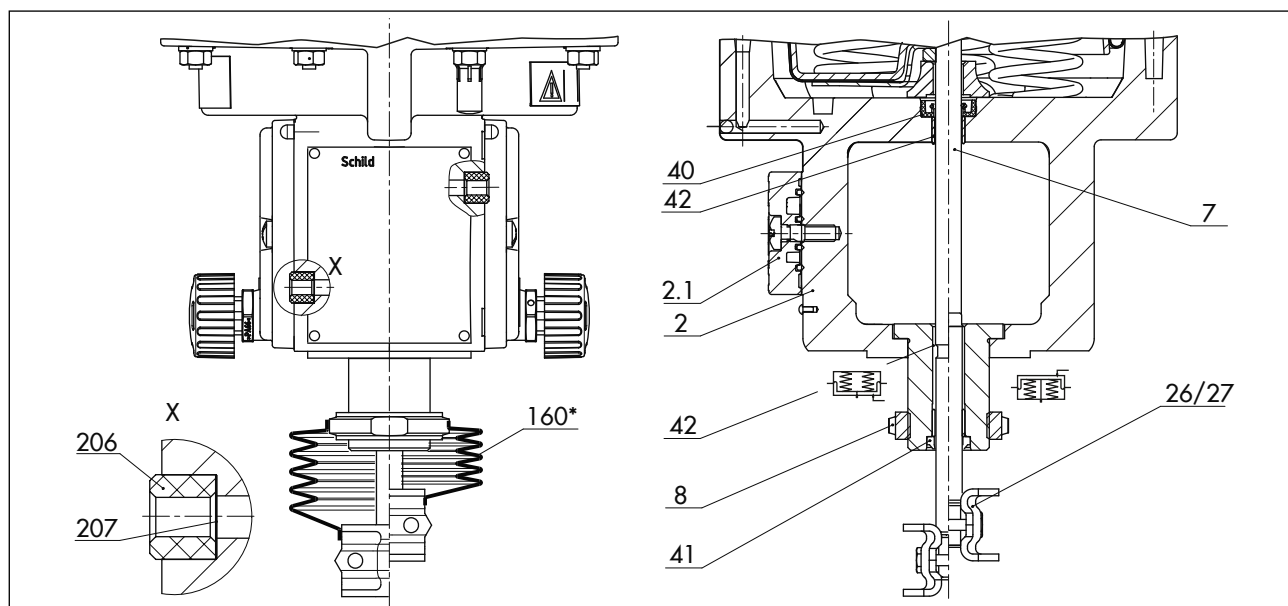
図 25: アクチュエータ タイプ 3277-5
