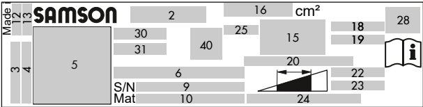
図 1: アクチュエータ タイプ 3271/3277 またはタイプ 2780（操作部面積 120 cm 2 ）の銘板の記載内容
