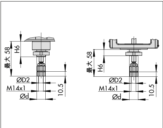
図 11: タイプ 3271-5 およびタイプ 3277-5、マイクロフロー弁 タイプ 3510 用の 7.5 mm トラベル付き
