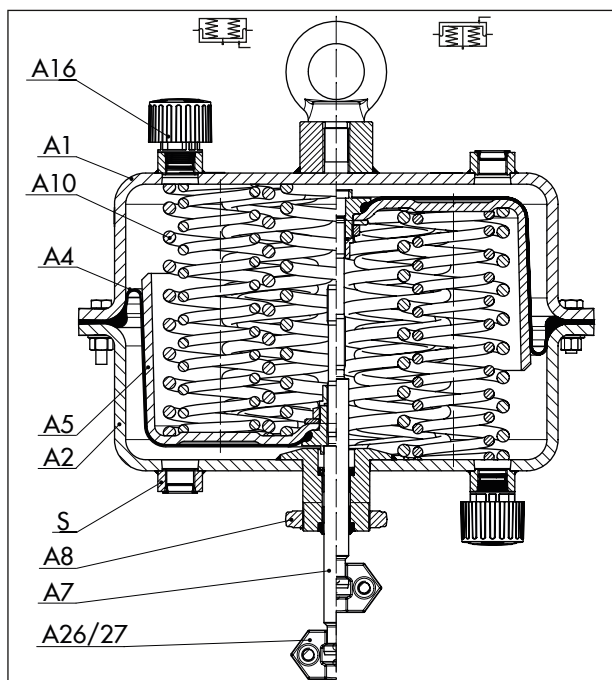
図 2: 空気式アクチュエータ タイプ 3271（操作部面積 1000 \text{ cm}^2 の例）
