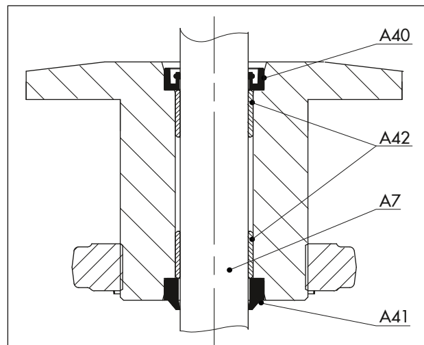
図 15: アクチュエータ軸シール（タイプ 3271）
