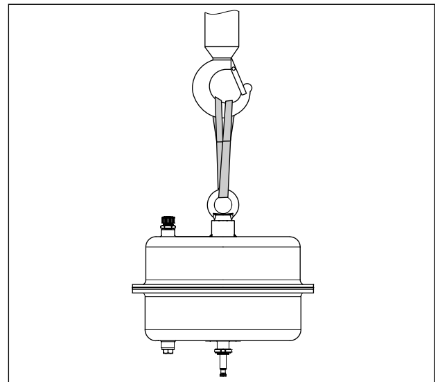
図 6: アクチュエータの吊上げポイント
