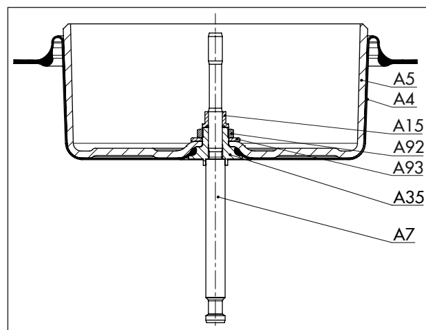
図 12: 「軸出」作動方向の場合の部品配列 (1000 cm 2 )
