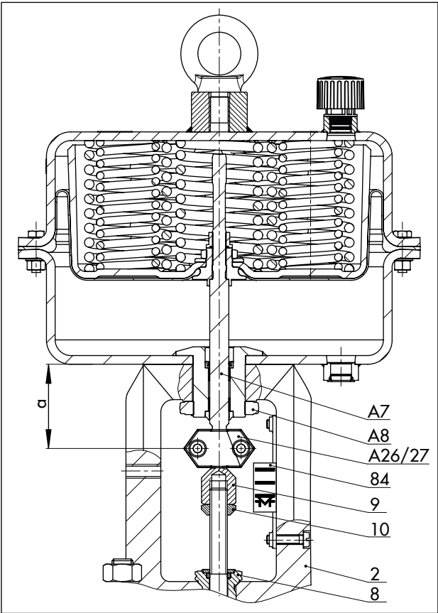
図 8: グローブ弁に取り付ける空気式アクチュエータ タイプ 3271
