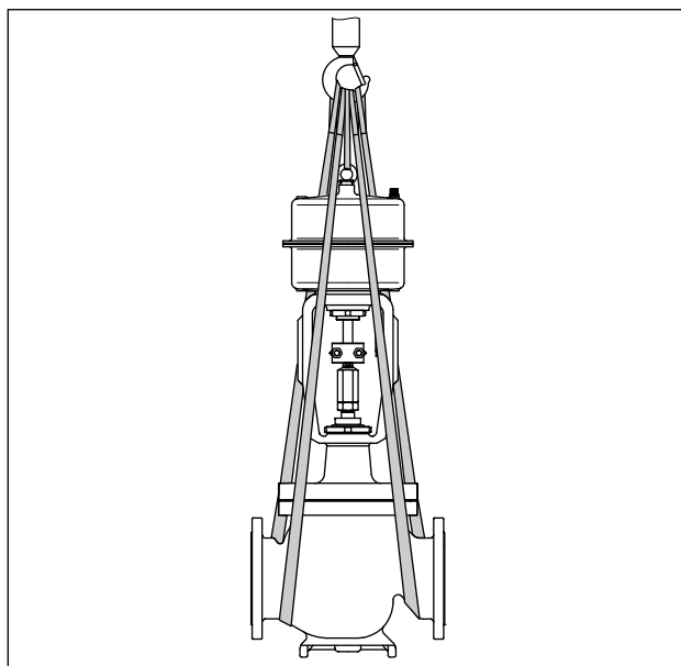
図 7: 調節弁の吊上げポイント（図は例）
