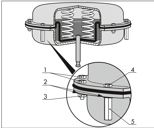
図 16: 事前に荷重がかけられたスプリング（構造図）
