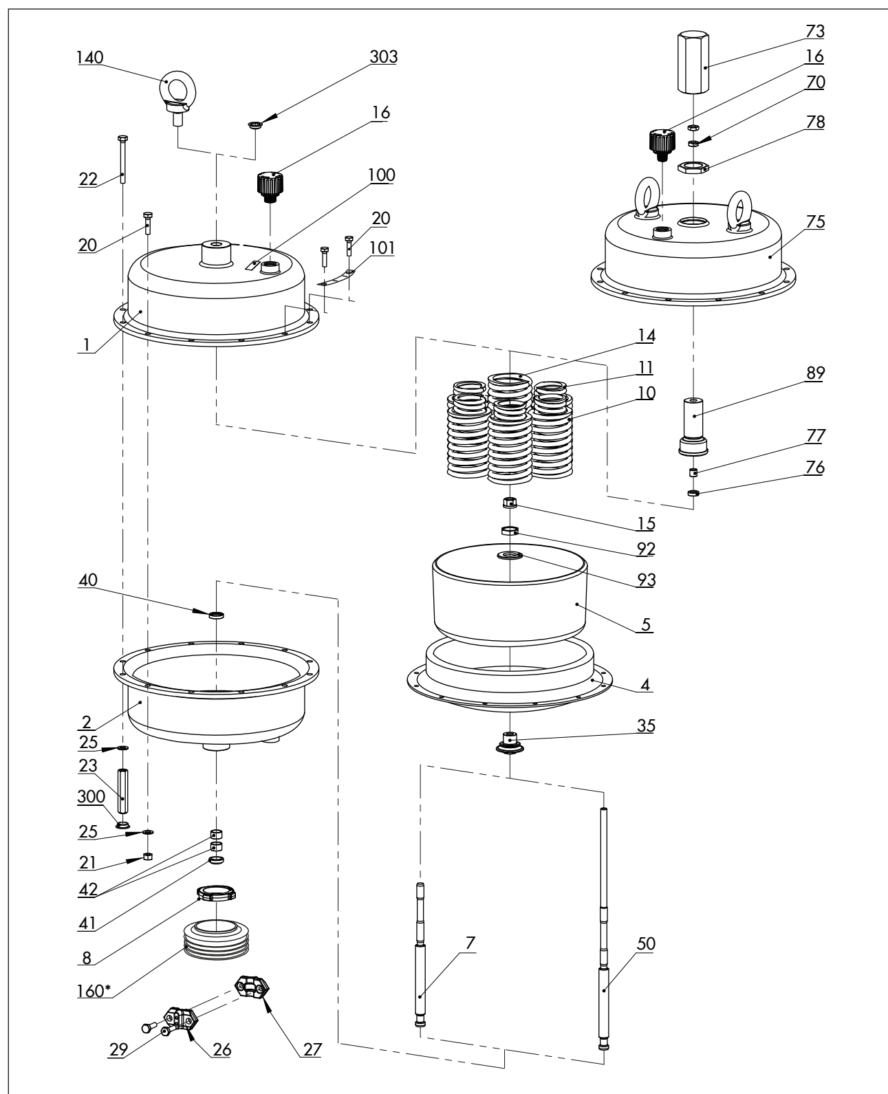
図 17: アクチュエータ タイプ 3271 (1000 cm 2 )
