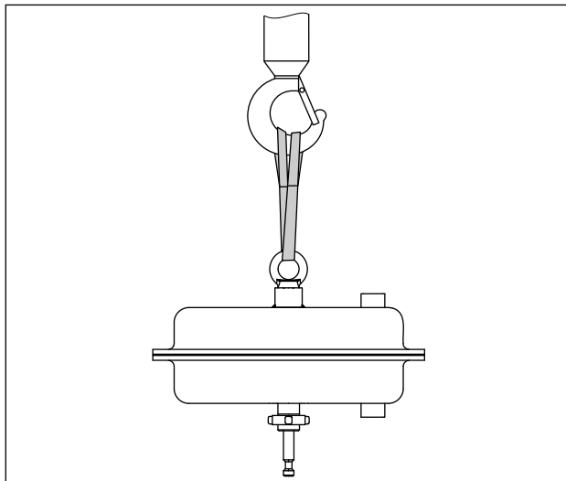
Rys. 6: Punkt podnoszenia w siłowniku
