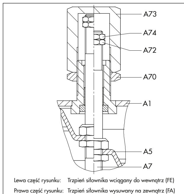
Rys. 11: Ogranicznik skoku
