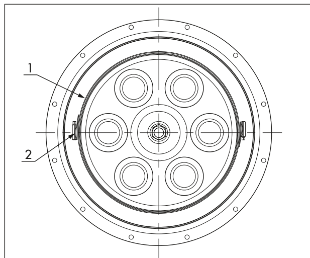
Rys. 14: Wyrównanie zamków zacisków z taśmą perforowaną
