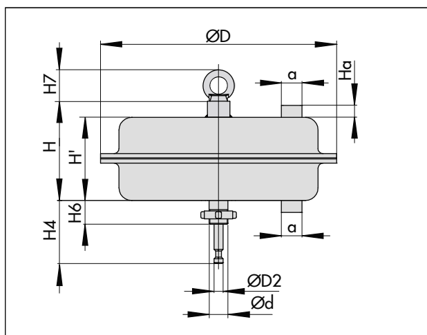
Rys. 3: Siłownik typu 3271 o powierzchni 1400-60 cm 2
