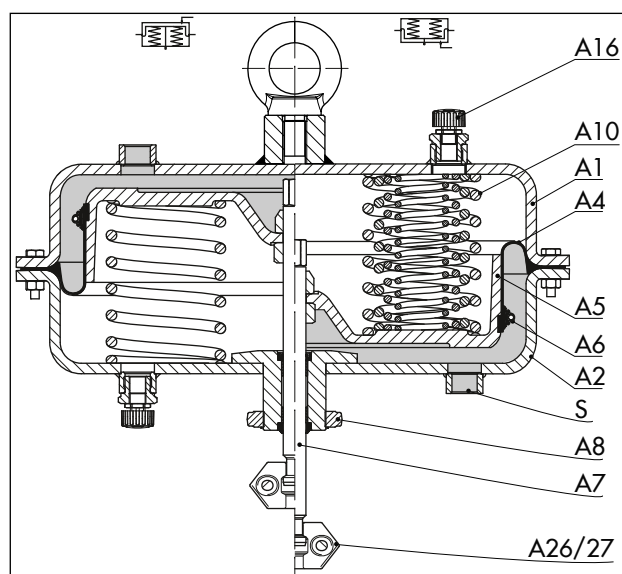
Rys. 2: Siłownik pneumatyczny typu 3271, na ilustracji wykonanie o powierzchni 1400-60 \text{ cm}^2
