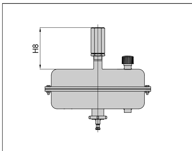
Rys. 4: Powierzchnia siłownika 1400-60 cm 2 , regulowany ogranicznik skoku
