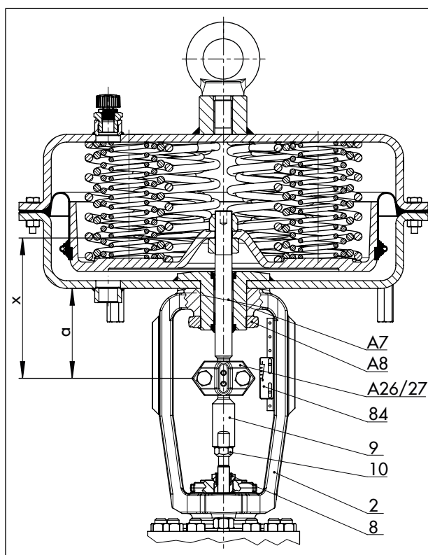
Rys. 8: Siłownik pneumatyczny typu 3271 zamontowany na zaworze skokowym
