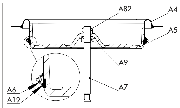
Rys. 13: Ułożenie części w siłowniku o kierunku działania „trzpień siłownika wysuwany na zewnątrz” (1400-60 cm 2 )
