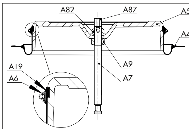
Rys. 15: Ułożenie części w siłowniku o kierunku działania „trzpień siłownika wciągany do wewnątrz” (1400-60 cm 2 )
