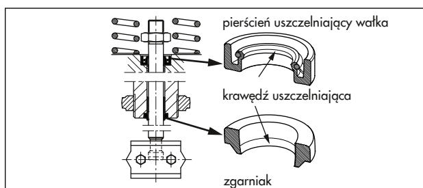
Rys. 16: Ułożenie pierścienia uszczelniającego wałek i zgarniaka.
