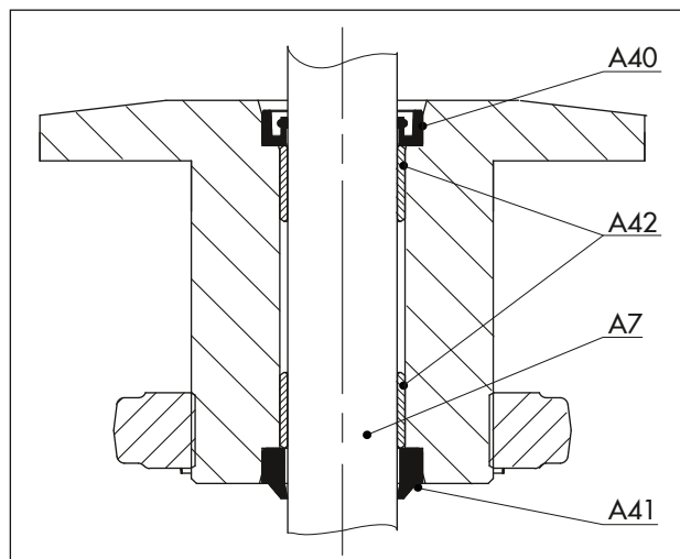
Rys. 17: Typ 3271 - uszczelka trzpienia siłownika
