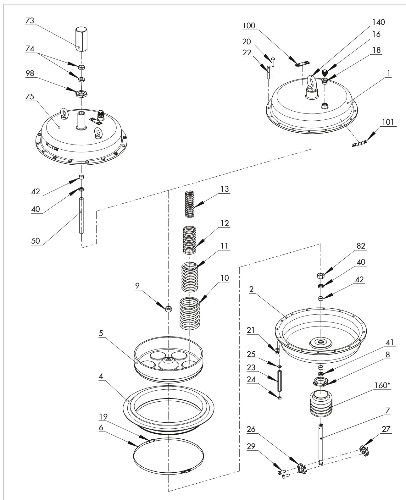
Rys. 19: Siłownik typu 3271, 1400-60 cm 2
