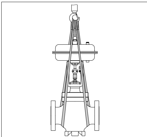
Rys. 7: Punkty podnoszenia w zaworze regulacyjnym (przykład)
