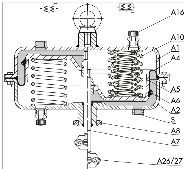
Rys. 12: Siłownik pneumatyczny typu 3271, na ilustracji wykonanie o powierzchni 1400-60 cm 2
