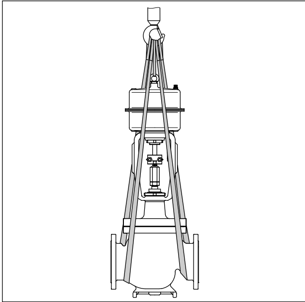
図 9: 調節弁の吊上げポイント（図は例）
