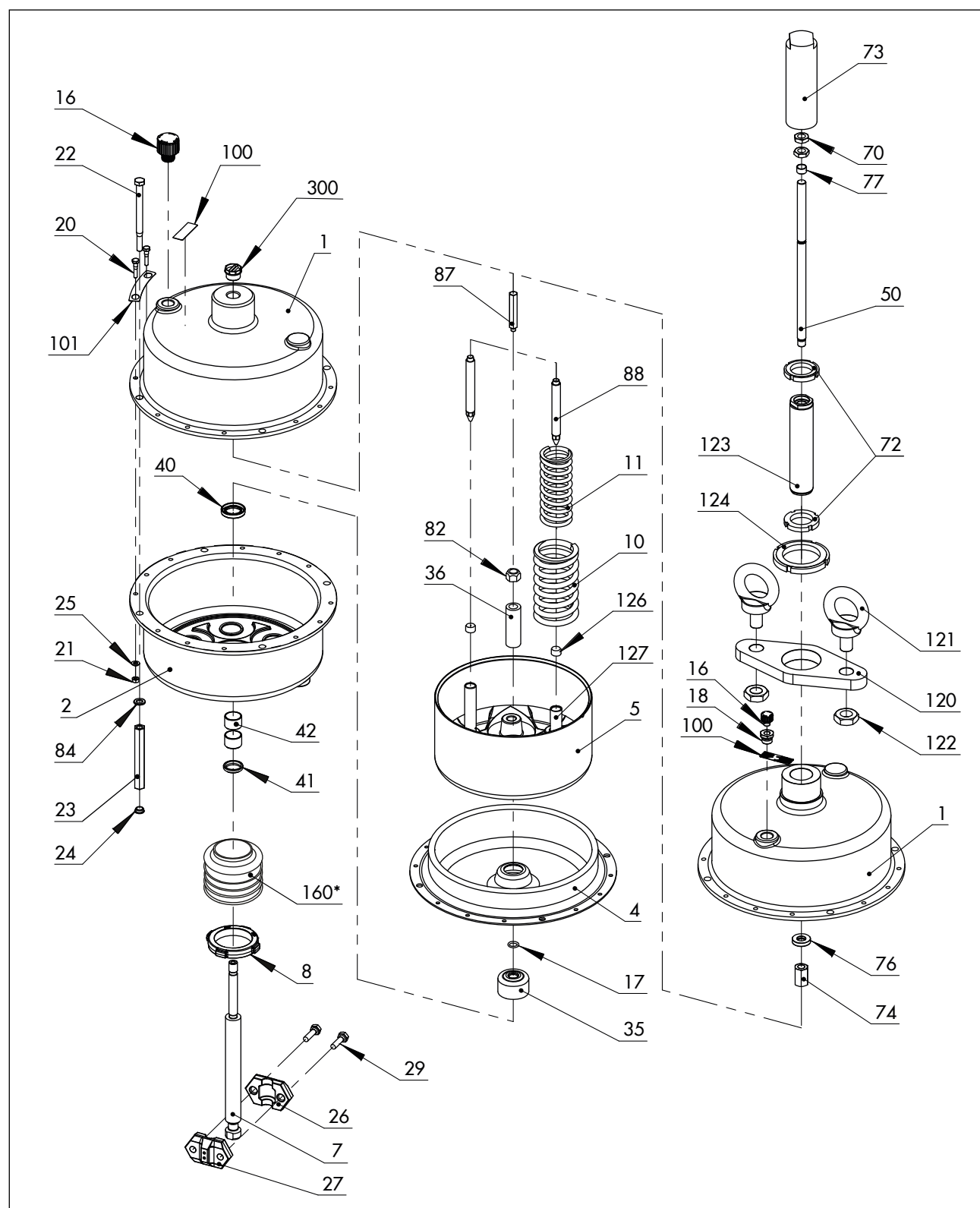
図 17: アクチュエータ タイプ 3271 (1400-120 cm 2 )
