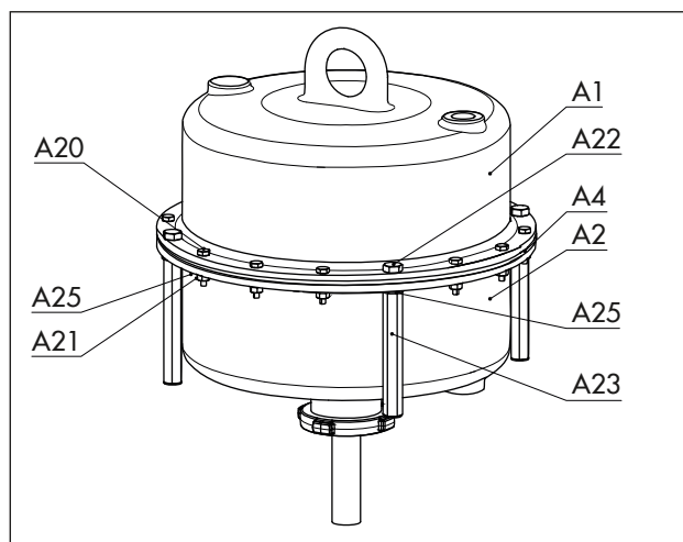
図 12: クランピングナットとボルト付きアクチュエータ
