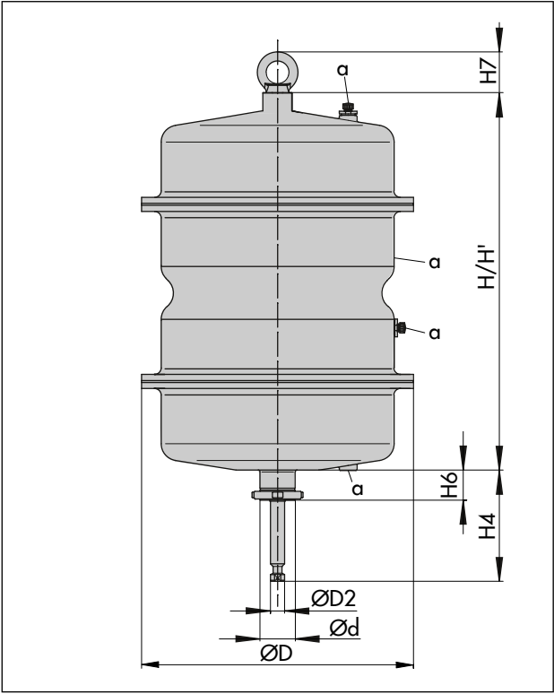
図 6: タイプ 3271、タンデムアクチュエータ
