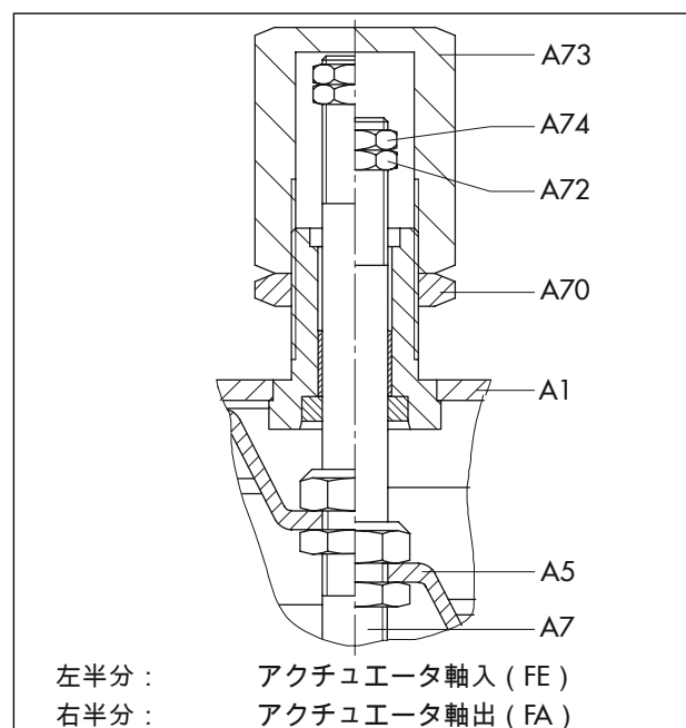
図 14: トラベルストップ
