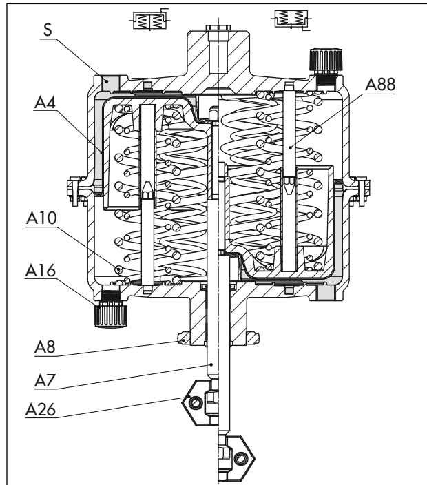
図 2: 空気式アクチュエータ タイプ 3271（操作部面積 1400\text{--}120 \text{ cm}^2 の例）
