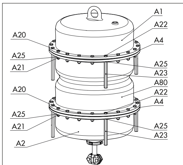
図 13: クランピングナットとボルト付きタンデムアクチュエータ
