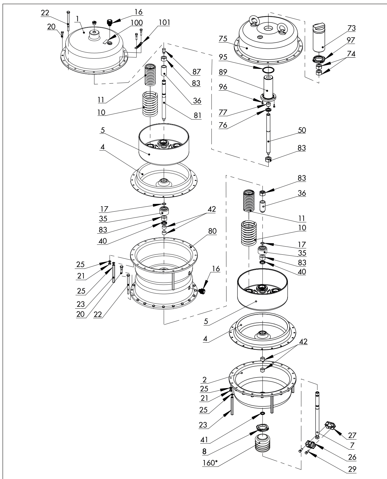
図 19: アクチュエータ タイプ 3271 (2x 2800 cm 2 )
