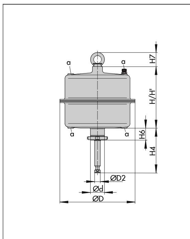
図 4: タイプ 3271、操作部面積 1400-120 cm 2
