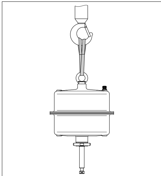
図 8: アクチュエータの吊上げポイント
