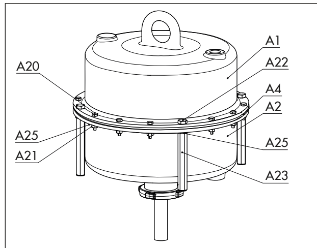
図 15: クランピングナットとボルト付きアクチュエータ
