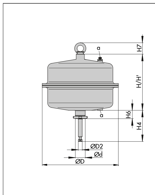
図 5: タイプ 3271、操作部面積 2800 cm 2
