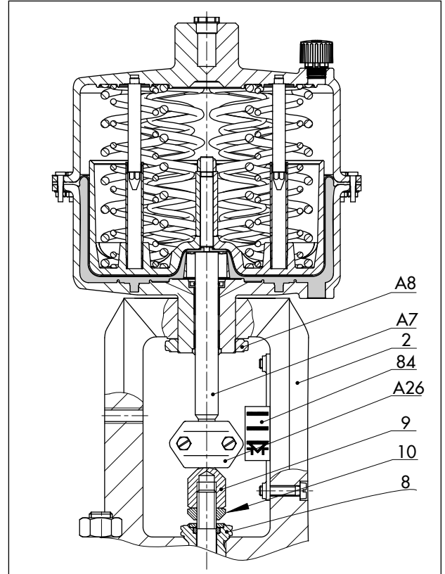
図 10: グローブ弁に取り付ける空気式アクチュエータ タイプ 3271
