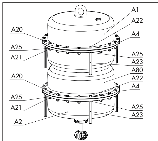
図 16: クランピングナットとボルト付きタンデムアクチュエータ
