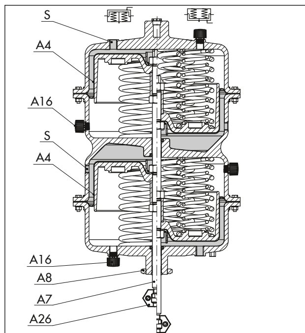
図 3: 空気式アクチュエータ タイプ 3271（操作部面積 2 \times 2800 \text{ cm}^2 の例）
