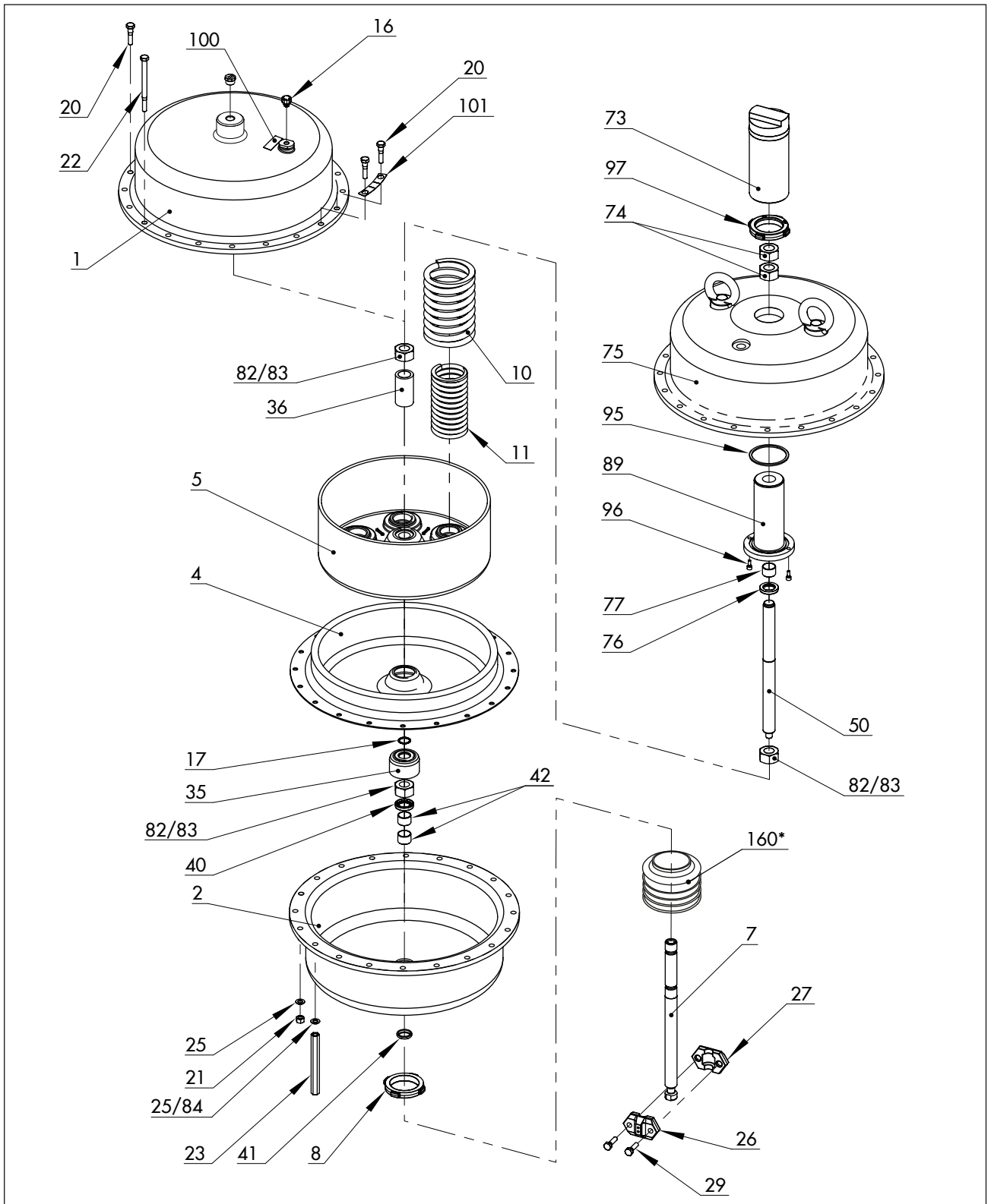
図 18: アクチュエータ タイプ 3271 (2800 cm 2 )
