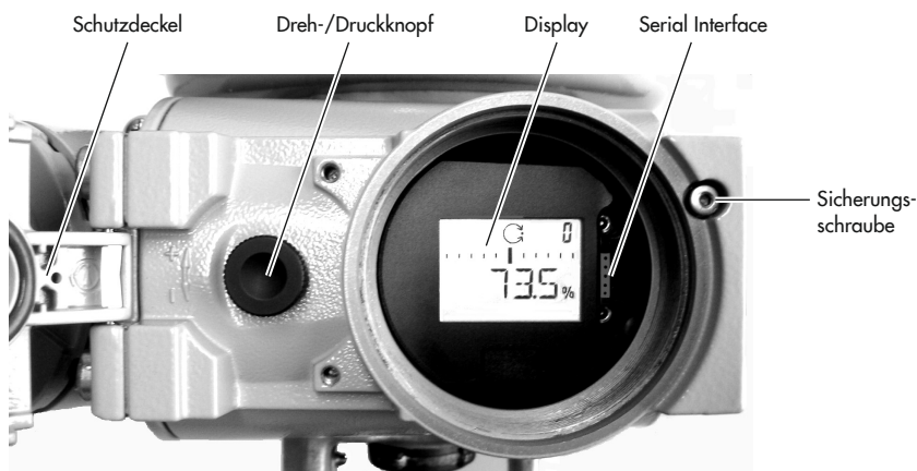
Bild 16: Bedienelemente des Stellungsreglers Typ 3731-3
