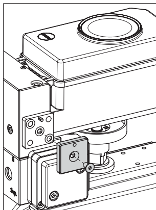
Fig. 5-18: Montage du sélecteur
