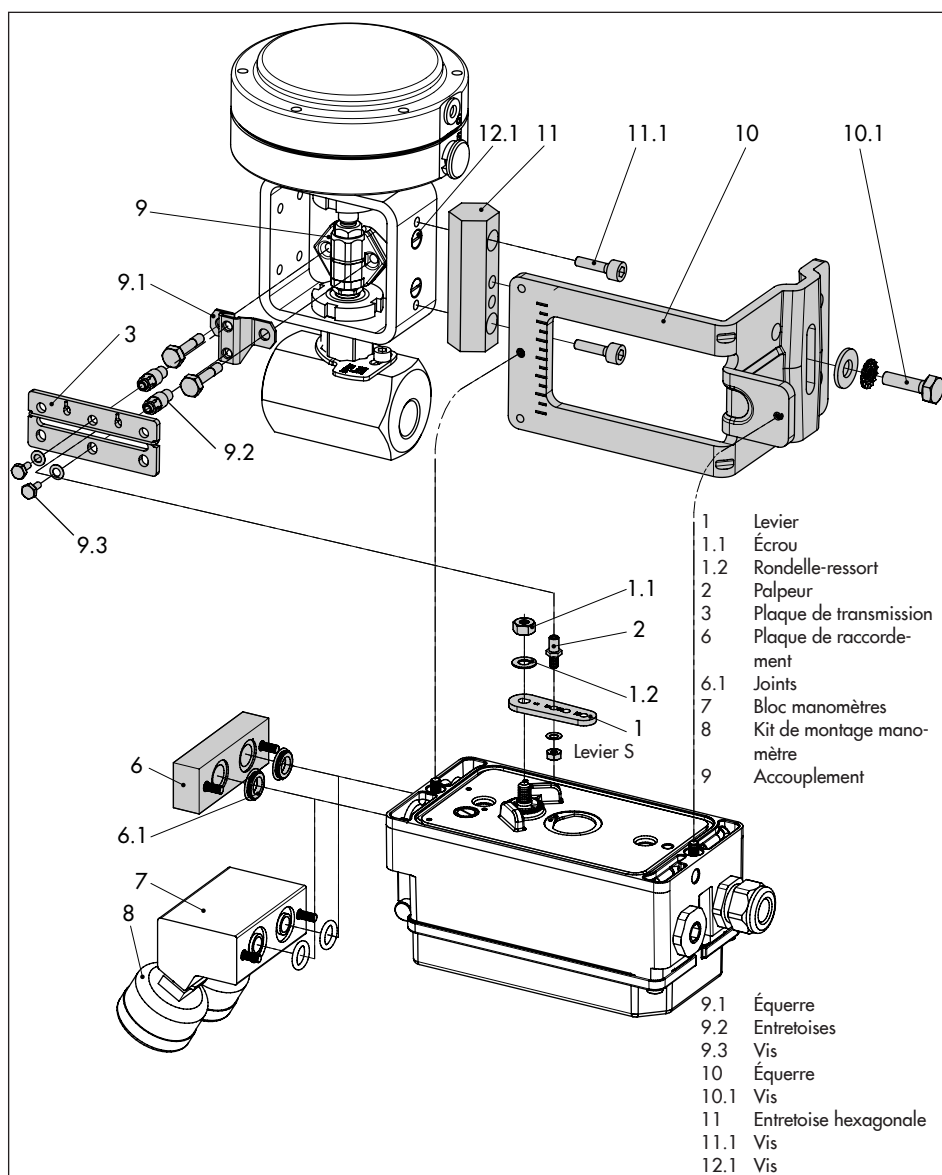
Fig. 5-11: Montage sur microvanne type 3510
