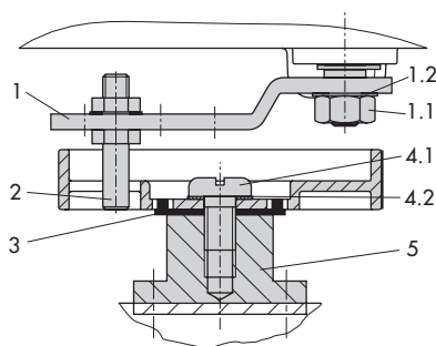
Fig. 5-22: Montage du disque d'accouplement sur un servomoteur type 3278
