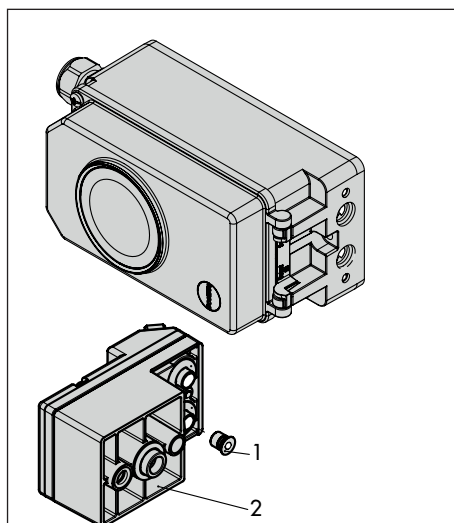
Fig. 5-6: Montage de la restriction de débit (1) sur le bloc de raccordement (2)
