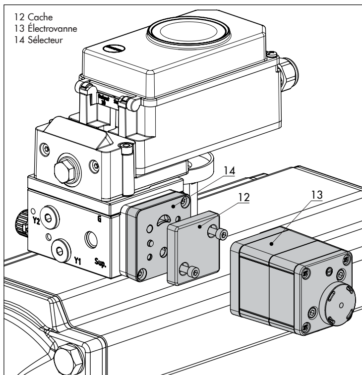
Fig. 5-21: Montage d'une électrovanne
