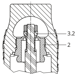
Clapet pour petits débits, C_v \leq 5 sans soufflet d'équilibrage
