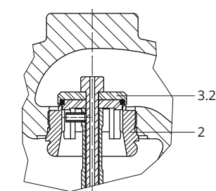
Clapet à étanchéité souple
