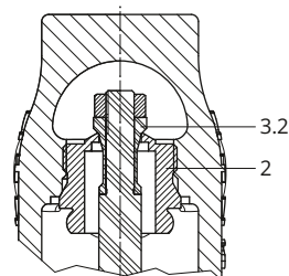
Clapet pour petits débits, C_v \leq 5 sans soufflet d'équilibrage
