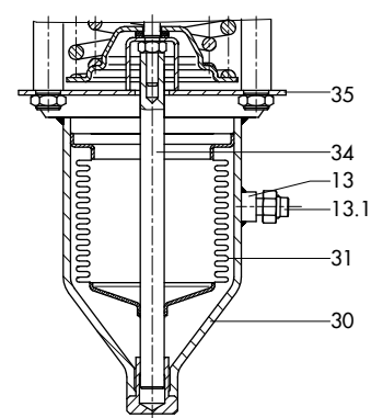
Servomoteur à soufflet : 200 à 600 kPa · 500 à 1000 kPa
