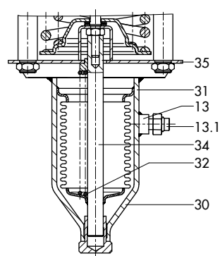
Servomoteur à soufflet : 1000 à 2200 kPa · 2000 à 2800 kPa
