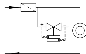
Einbau in Kurzschlussleitung
