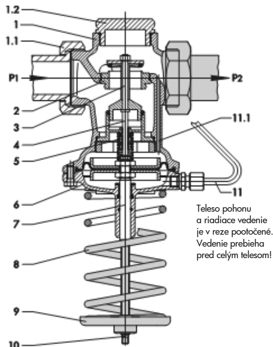
Typ 45-6, DN 15 do 50 s maticami a navarovacími koncami
