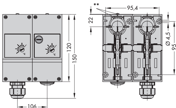
Termostato doppio STW/STB Tipo 5349
