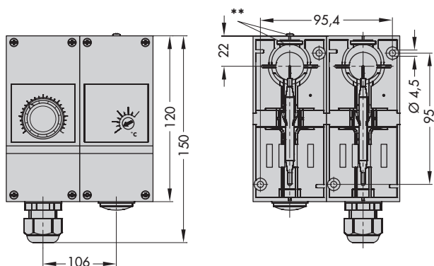
Termostato doppio TR/STW Tipo 5348
