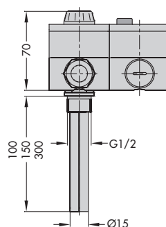
Dimensioni con pozzetto (accessori)
