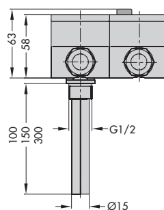
Dimensioni con pozzetto (accessori)
