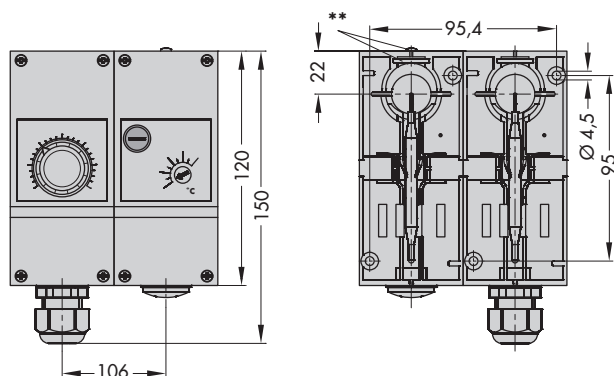
Termostato doppio TR/STB Tipo 5347
