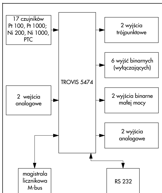
Rys. 2 · Wejścia i wyjścia regulatora
