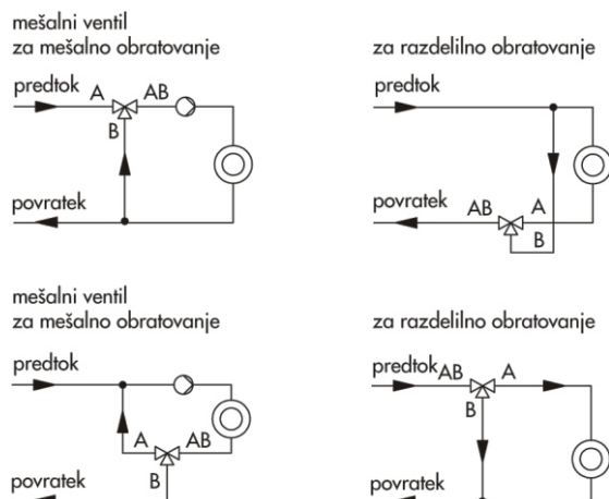
Slika 5 Primeri vgradnje
