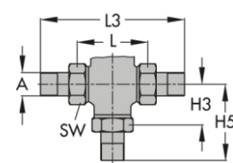
Izvedba z zunanjim navojem ter navojno spojko in privojnimi nastavki
