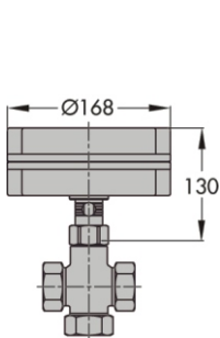
Tip 3226/2780-1: DN 15 do 50
