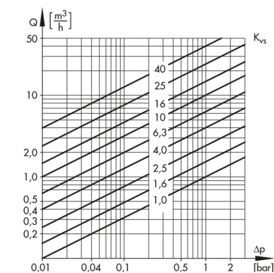
Slika 6 Diagram volumnskega pretoka za vodo
