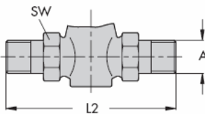
Menetes végekkel rendelkező kivitel
