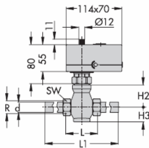
Típus 3222/5857: DN 15 ... 25 Hegeszthető toldatos kivitel
