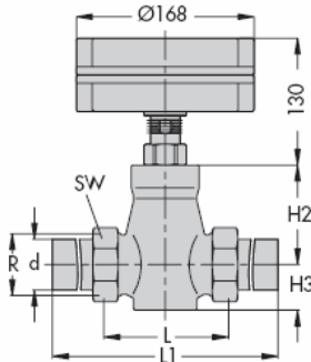
Típus 3222/2780-1: DN 15 ... 50 Hegeszthető toldatos kivitel
