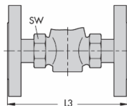
Karimás kivitel
