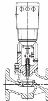
3. ábra · Típus 3241/3374 villamos állítószelep Típus 3374 villamos állítóművel és Típus 3241 átmeneti szeleppel
