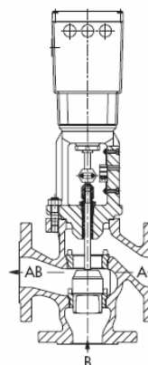
4. ábra · Típus 3244/3374 villamos állítószelep Típus 3374 villamos állítóművel és Típus 3244 háromjáratú szeleppel, keverőszelepként
