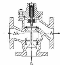
5. ábra · Típus 3244 háromjáratú szelep, elosztószelepként
