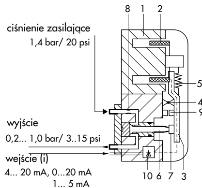
Rys. 4 · Schemat działania modułu przetwornika i/p typu 6112-02
