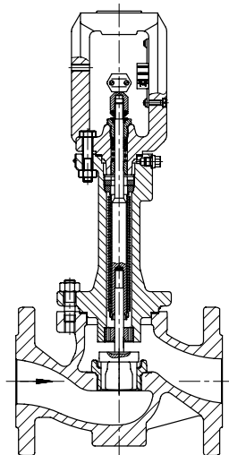
5. ábra · 241 típusú szelep, fém csőmembrántömítéssel
