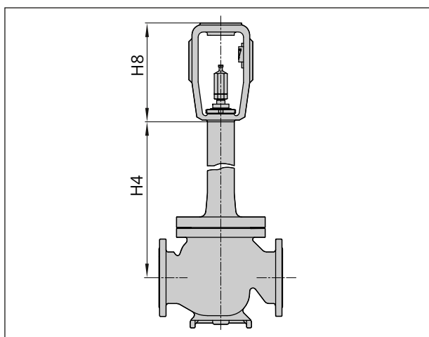
Fig. 8: Typ 3241 med isolerande del eller bälgtätning DN 200/NPS 8 och större
