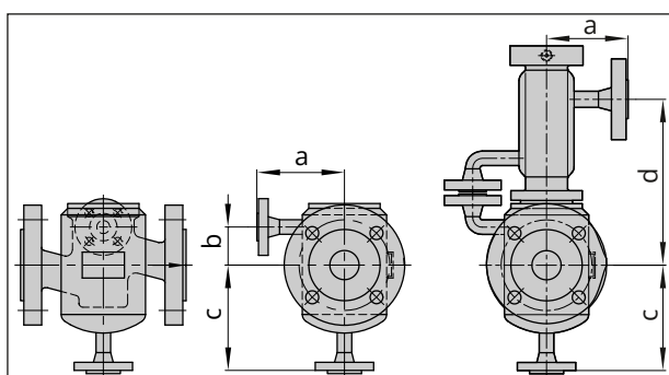
Fig. 9: Typ 3241 med värmejacka, upp till nominell storlek DN 100/NPS 4 · med isolerande del eller bälgtätning (höger)
