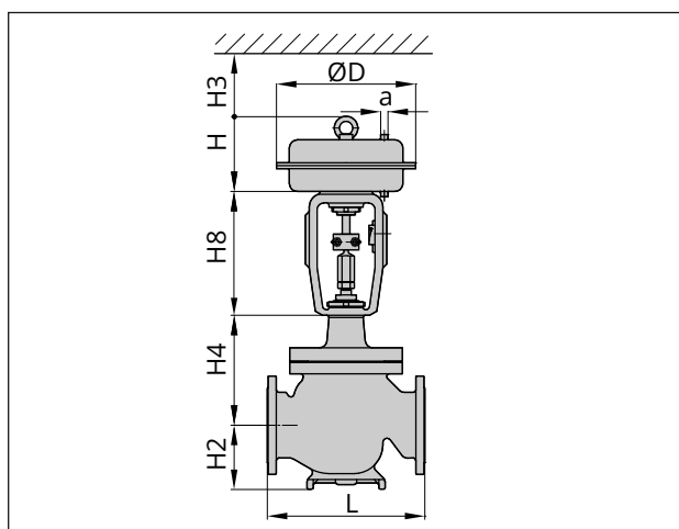
Fig. 4: Tipo 3241-1 (accionamiento neumático Tipo 3271) con paso nominal hasta DN 200/NPS 8
