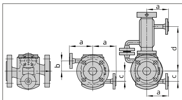
Fig. 9 : Type 3241 avec chemise de réchauffage à partir du diamètre nominal DN 150/NPS 6 · à droite dans la figure, avec pièce d'isolement/soufflet
