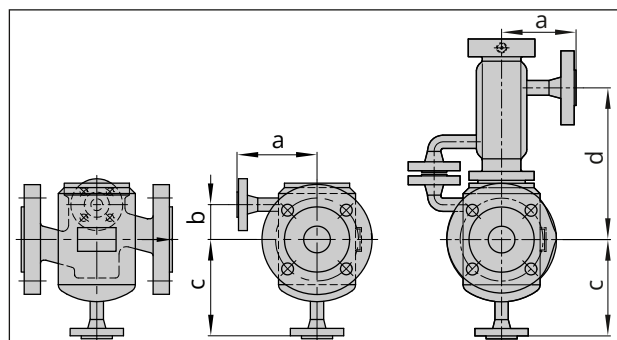
Fig. 8 : Type 3241 avec chemise de réchauffage jusqu'au diamètre nominal DN 100/NPS 4 · à droite dans la figure, avec pièce d'isolement/soufflet
