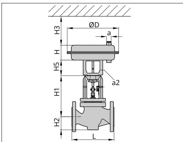
Fig. 5 : Type 3241-7 (servomoteur pneumatique type 3277) jusqu'au diamètre nominal DN 150/NPS 6/DN 150A
