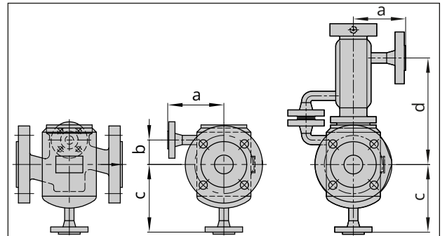
Fig. 8: Tip 3241, ısıtma ceketli, DN 100/NPS 4 nominal boyutuna kadar · İzolasyon bölümlü veya metal körüklü salmistrallı (sağ)
