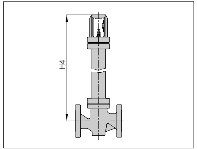
Fig. 6: Tip 3241 izolasyon bölümlü veya metal körüklü salmistrallı, DN 150/NPS 6/DN 150A nominal boyutuna kadar
