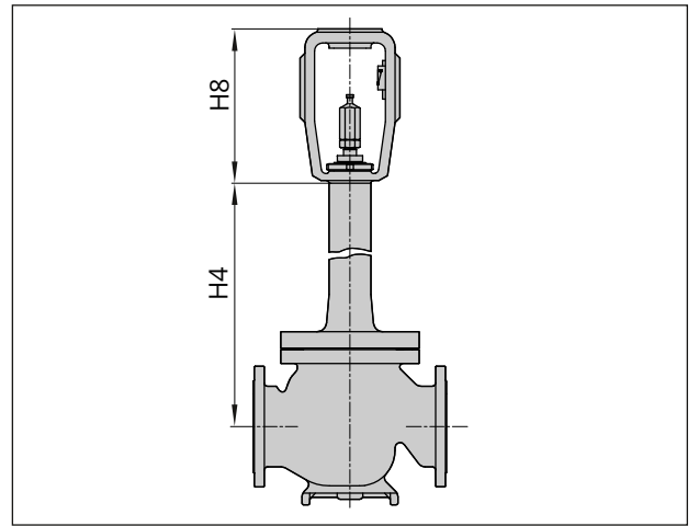
Fig. 7: Tip 3241 izolasyon bölümlü veya metal körüklü salmistrallı, DN 200/NPS 8 ve daha büyük
