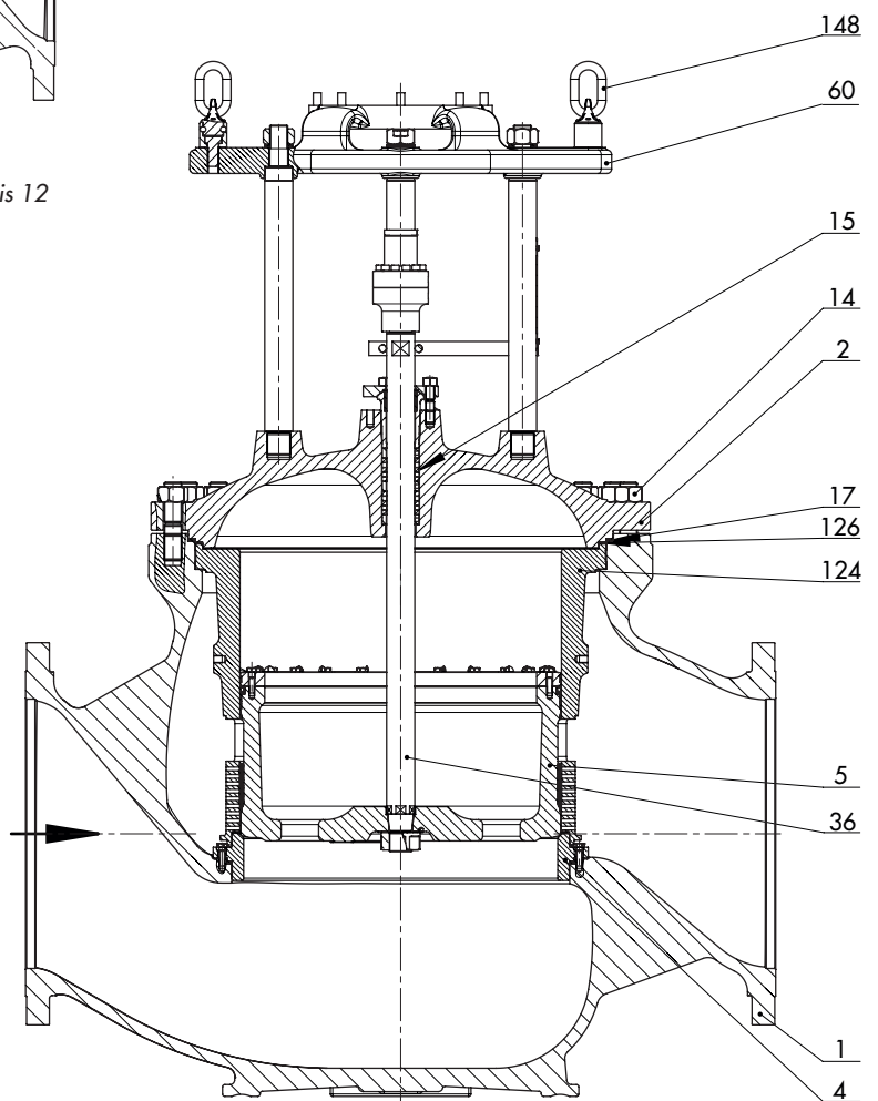
Bild 4: Typ 3591 mit geflanschem Sitz · NPS 16 bis 28 (Class 300 bis 900)
