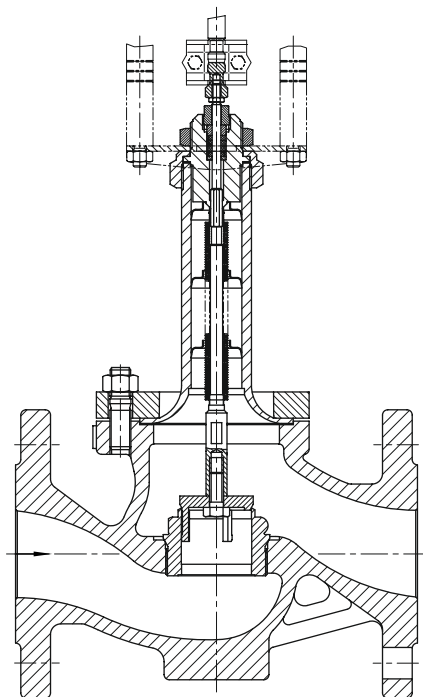
Bild 5: Durchgangsventil Typ 3531-IP für Wärmeträgeröl in NPS ½ bis 2
