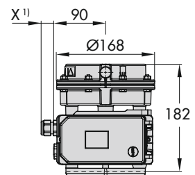
Typ 3372 mit Stellungsregler Bauart 3730
