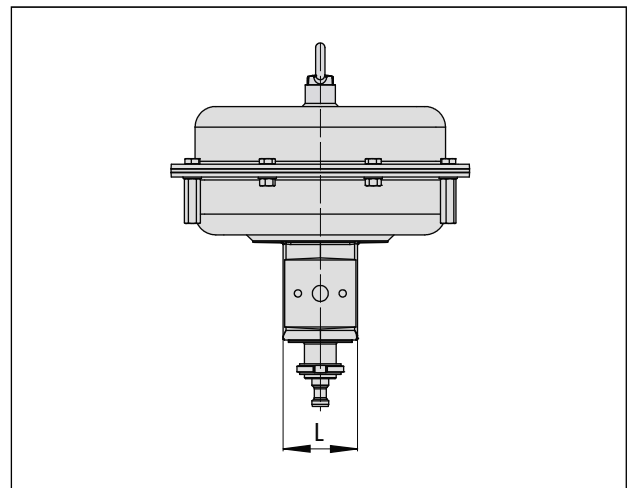
図 23: タイプ 3277 ヨーク付き（側面図）・操作部面積 750v2 cm 2
