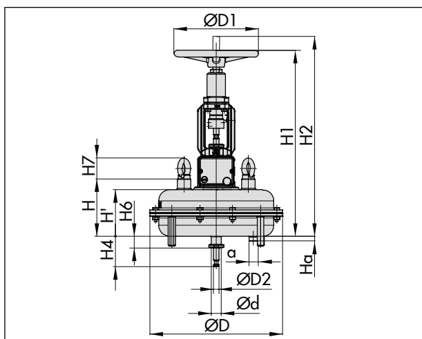
図 18: 空気式アクチュエータ タイプ 3271、手動ハンドルとトラベルストップを両サイドに装備
