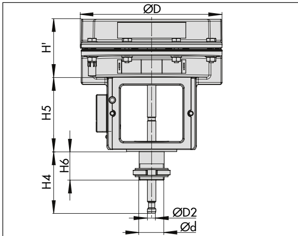
図 20: タイプ 3277-5 ・操作部面積 120 cm 2
