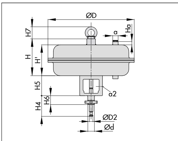
図 22: タイプ 3277、ヨーク付きで付属品の直接接続に対応 ・操作部面積 750v2 cm 2
