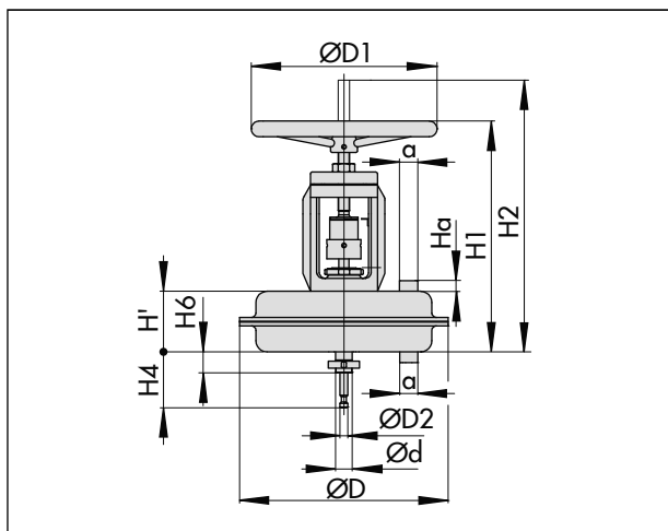
図 17: タイプ 3271 追加の手動ハンドル付き
