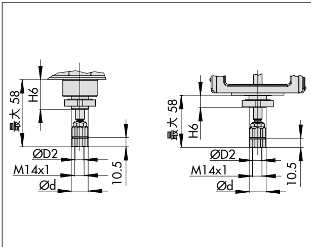
図 27: タイプ 3271-5 およびタイプ 3277-5、マイクロフロー弁 タイプ 3510 用の 7.5 mm トラベル付き
