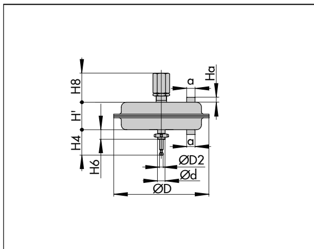
図 19: タイプ 3271 トラベルストップ付き
