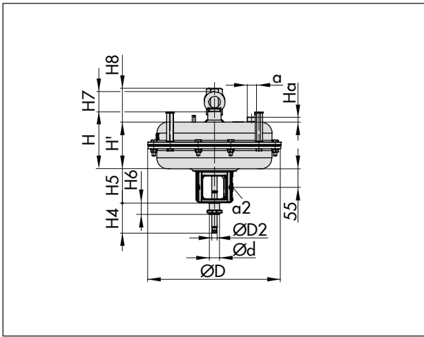
図 26: タイプ 3277 トラベルストップ付き
