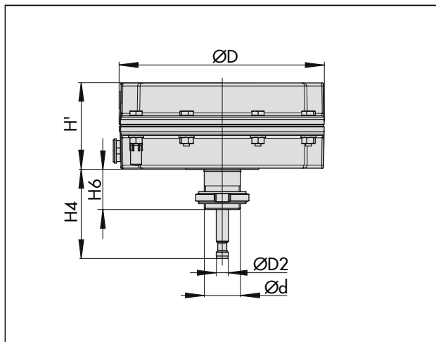
図 14: タイプ 3271-5 ・ 操作部面積 120 cm 2
