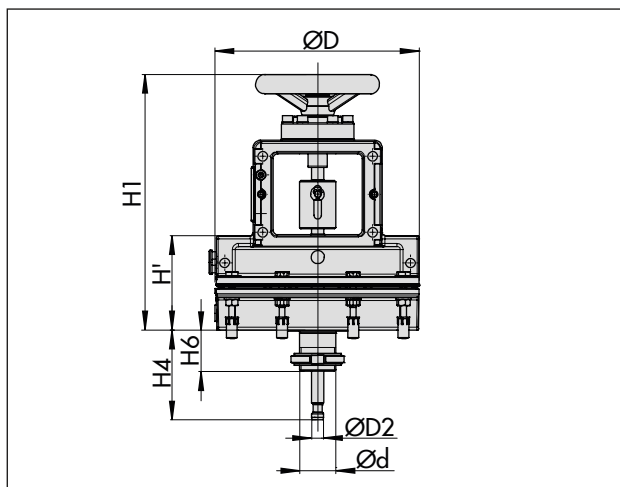
図 15: タイプ 3271-5 追加の手動ハンドル付き
