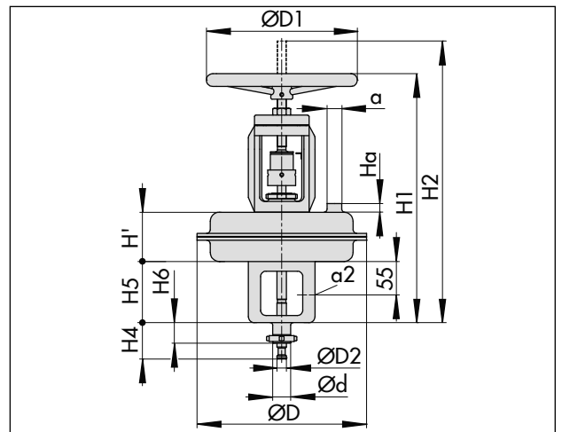
図 24: タイプ 3277 追加の手動ハンドル付き
