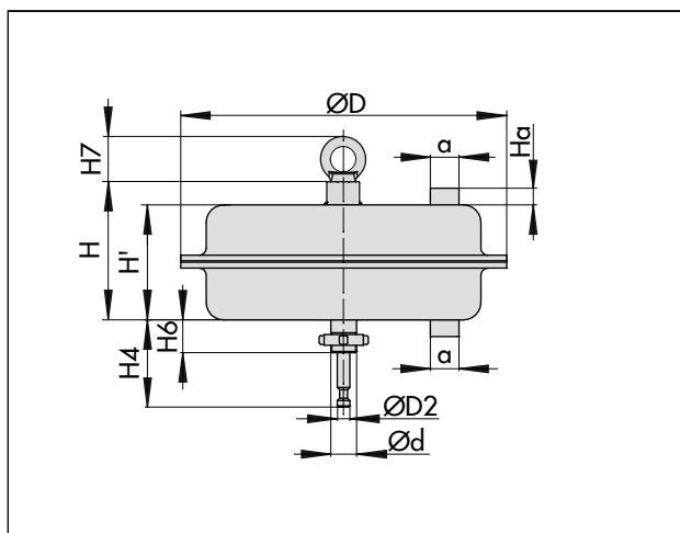
図 16: タイプ 3271、操作部面積 750v2 cm 2
