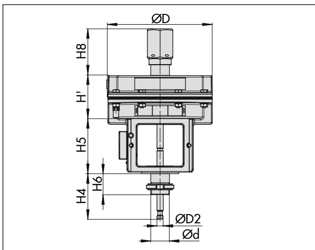
図 21: タイプ 3277-5 トラベルストップ付き
