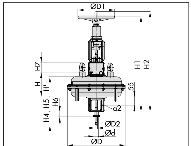
図 25: 空気式アクチュエータ タイプ 3277、手動ハンドルとトラベルストップを両サイドに装備
