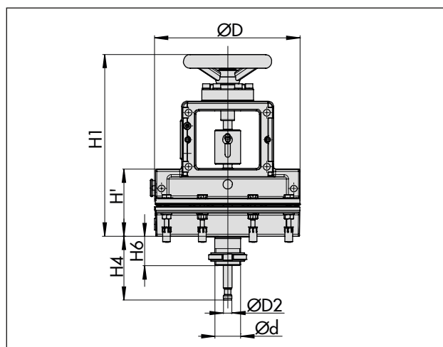
Fig. 16: Typ 3271-5 med extra handhjul
