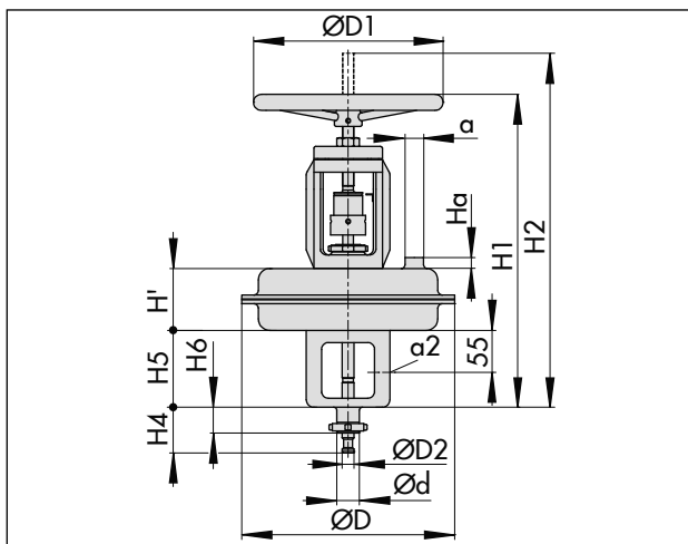
Fig. 25: Typ 3277 med extra handhjul
