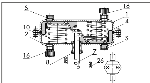
Fig. 7: Typ 3271 · Höger: med extra fjädrar
