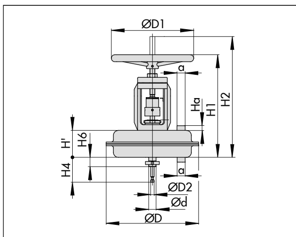
Fig. 18: Typ 3271 med extra handhjul
