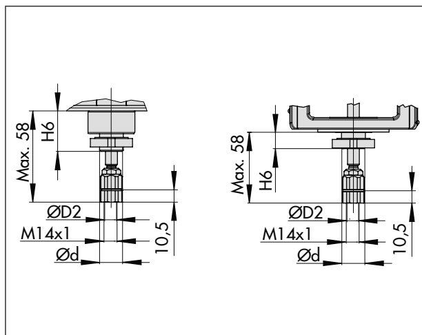
Fig. 28: Typerna 3271-5 och 3277-5 med 7,5 mm slaglängd för mikroflödesventil av typen 3510
