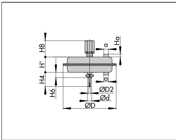
Fig. 20: Typ 3271 med slaglängdsstopp
