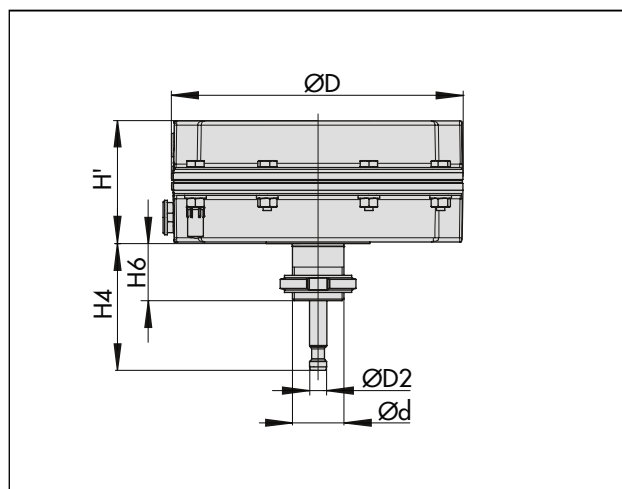
Fig. 15: Typ 3271-5 · 120 cm 2 ställdonsområde
