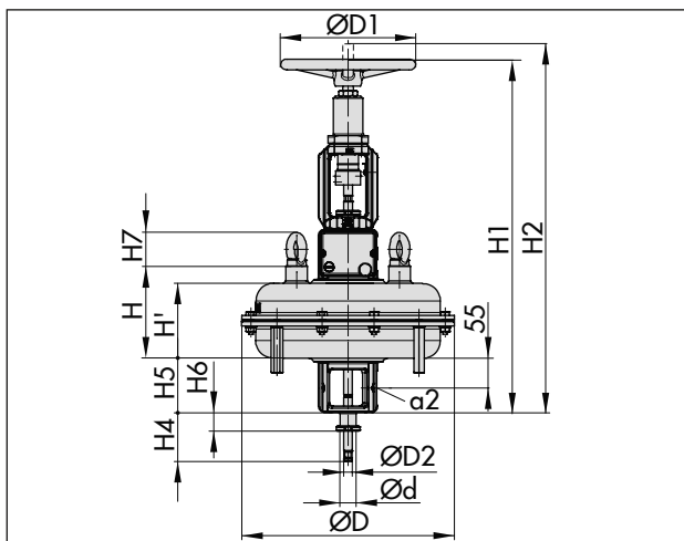
Fig. 26: Pneumatiskt ställdon av typen 3277 med handhjul och slaglängdsstopp på båda sidor
