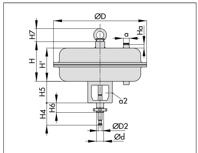
Fig. 23: Typ 3277 med ok för direktfäste av tillbehör · 750v2 cm 2 ställdonsområde
