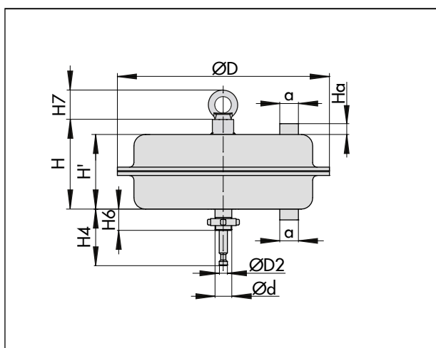
Fig. 17: Ställdon typ 3271 med 750v2 cm 2 ställdonsområde
