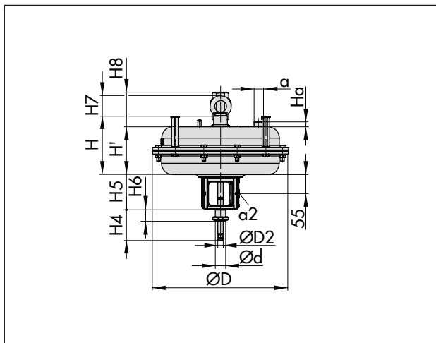
Fig. 27: Typ 3277 med slaglängdsstopp
