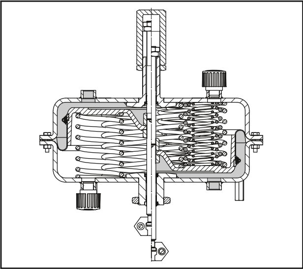
Fig. 3: Ejecución 1400-60 cm² con limitador de carrera ajustable en ambos lados
