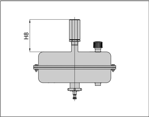
Fig. 5: Superficie de accionamiento 1400-60 cm 2 , con limitación de carrera ajustable
