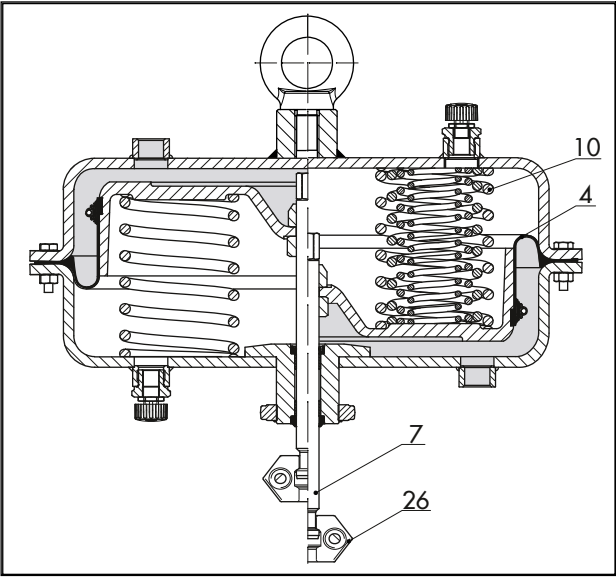
Fig. 2: Tipo 3271, 1400-60 cm² · Mitad izquierda: sentido de actuación FE · Mitad derecha: sentido de actuación FA
