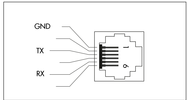
Bild 23: Belegung der RJ-12-Buchse
