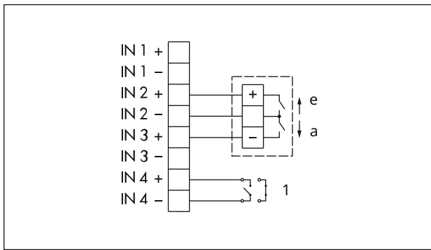
Bild 19: Anschlussbelegung bei Applikation Dreipunkt mit Dreidraht-Anschluss
