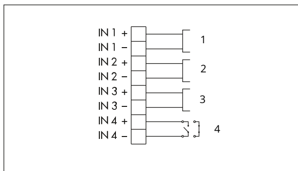
Bild 17: Anschlussbelegung bei Applikation PID-Regler - Temperaturregelung
