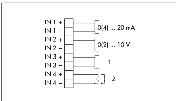
Bild 20: Anschlussbelegung bei Applikation Temperaturregelung bei Eingangssignalausfall
