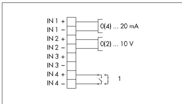
Bild 15: Anschlussbelegung bei Applikation Stellungsregler
