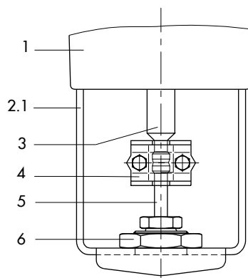
Bild 5: Anbau · Ausführung mit integriertem Joch
