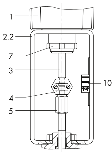
Bild 10: Anbau an Typ 3214
