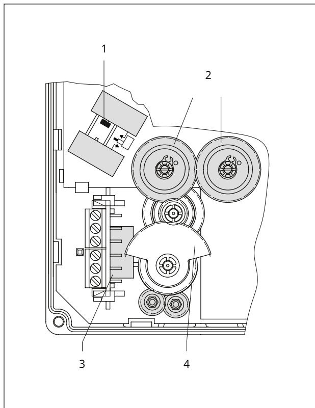
Bild 3: Teilansicht bei geöffnetem Deckel · Typ 3374
