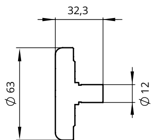
Bild 28: Maße in mm · Handrad als Sonderausführung
