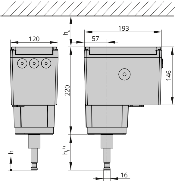
Bild 25: Maße in mm · Typ 3374-15, -17, -26 und -36, (Form A)
