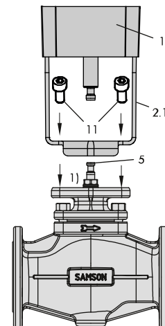
Bild 6: Anbau · Ausführung mit Antriebsjoch und Zubehör V2001
