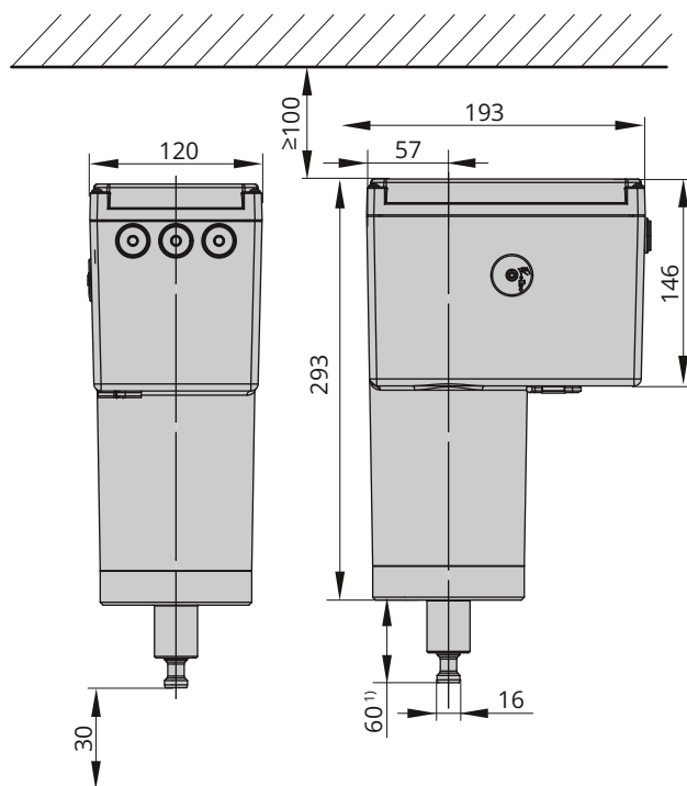
Bild 27: Maße in mm · Typ 3374-35, Ausführung Form A
