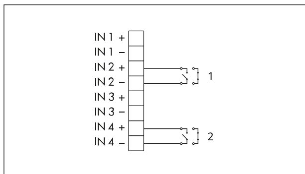
Bild 18: Anschlussbelegung bei Applikation Auf/Zu-Betrieb
