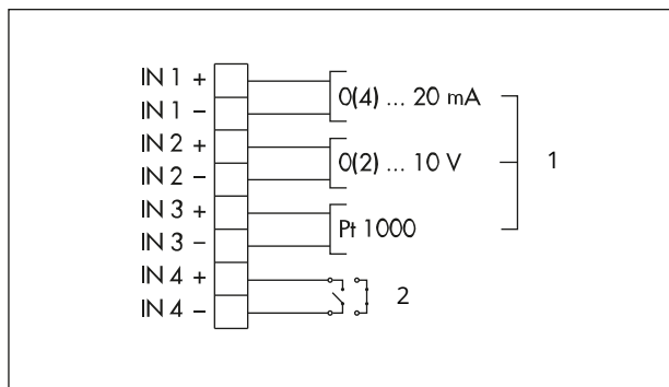
Bild 16: Anschlussbelegung bei Applikation PID-Regler
