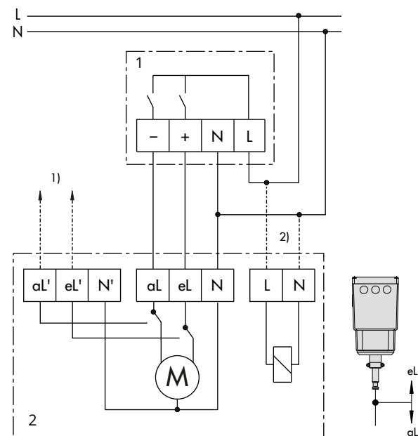
Bild 11: Elektrischer Anschluss
