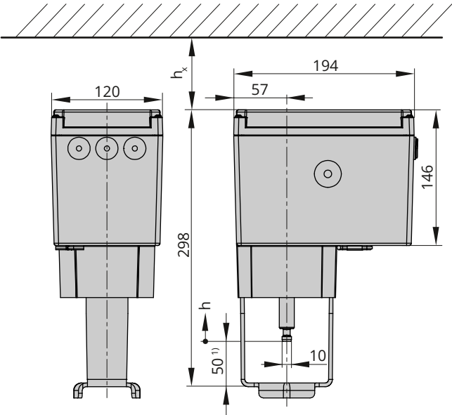
Bild 24: Maße in mm · Typ 3374-10, -11, -21 und -31 (Form B)
