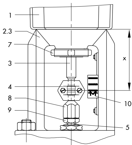
Bild 9: Anbau an Ventil Bauart 240
