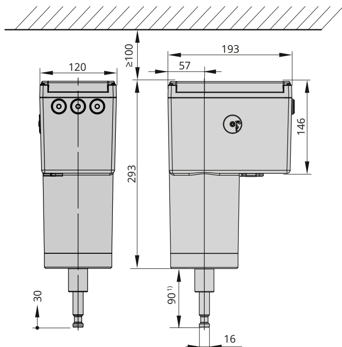
Bild 26: Maße in mm · Typ 3374-25 und -27, Ausführung Form A
