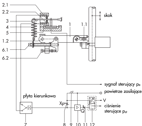
Rys. 6 · Schemat działania ustawnika pozycyjnego typu 3766 (połączenie przegubowe dźwigni odczytującej przy montażu na siłowniku pneumatycznym typu 3277)
