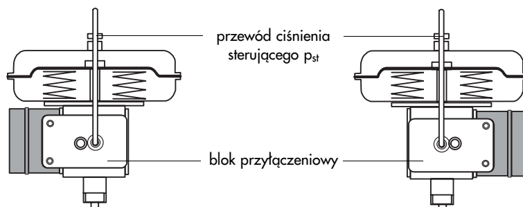
Rys. 11.3 · Kierunek działania << montaż z lewej strony
