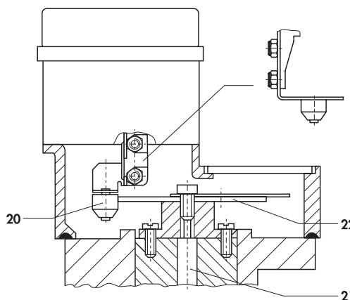
Rys. 8 · Przenoszenie ruchu obrotowego do ustawnika pozycyjnego
